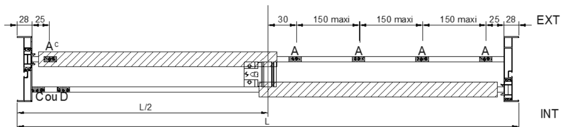
BI-RAILS 2 VANTAUX
