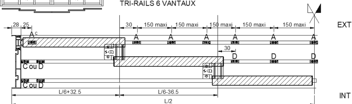
TRI-RAILS 6 VANTAUX
