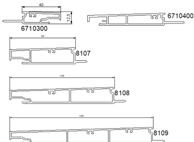
Pièces d'appui
