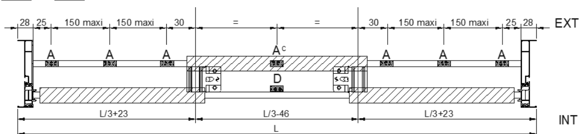
BI-RAILS 3 VANTAUX INDEPENDANTS - VTL SERVICE INT
