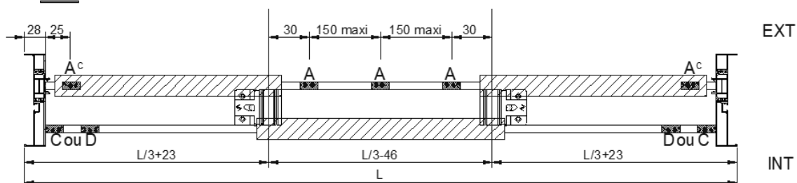
BI-RAILS 3 VANTAUX INDEPENDANTS - VTL SERVICE EXT
