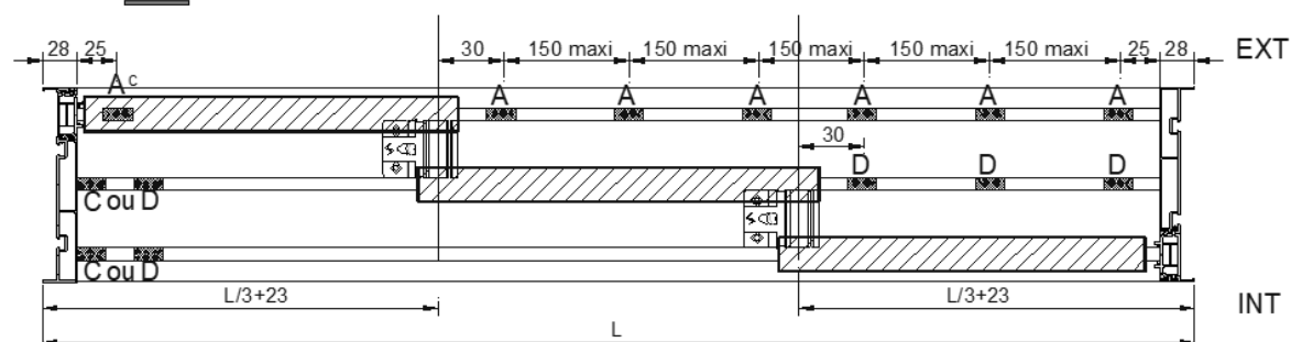
TRI-RAILS 3 VANTAUX
