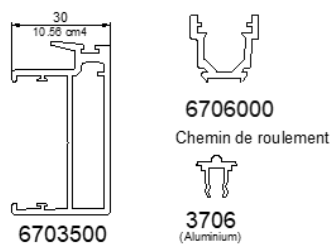
Autres profilés
