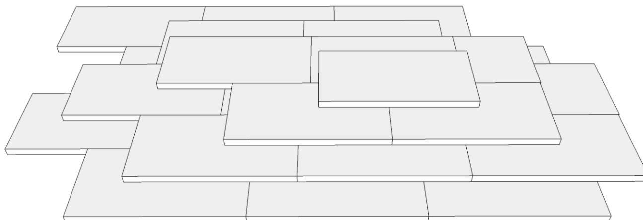
Figure 2 : Schéma de principe de la pose des différents lits des panneaux isolants en quinconce
