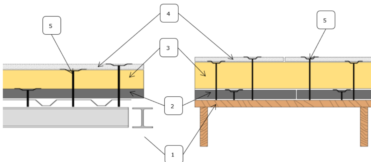
Figures 3 : Coupe de principe de la mise en œuvre de l'écran thermique et des panneaux isolants
