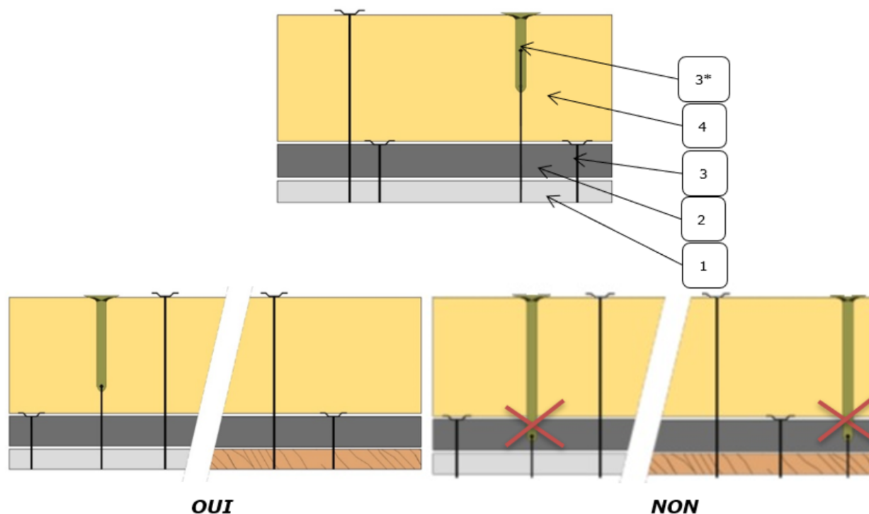
Figures 1 : Schéma de principe de l'utilisation des fixations mécaniques à rupteur de pont thermique
