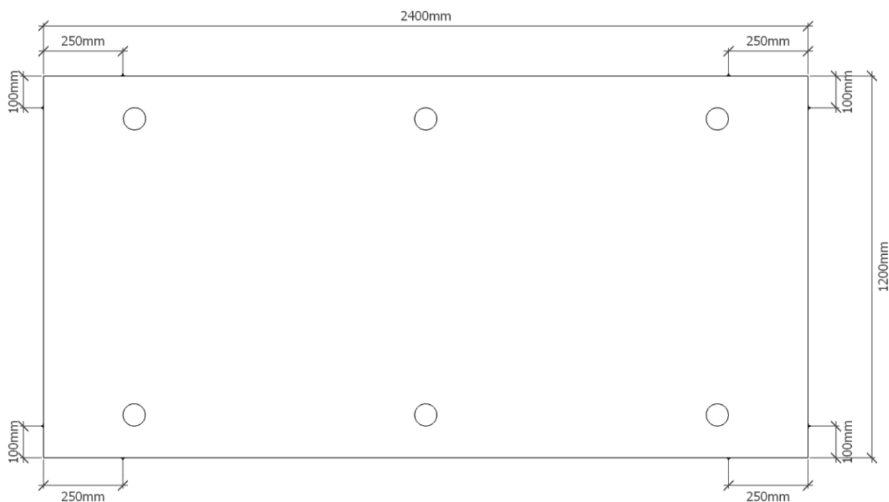
Figure 4.a – Fixations mécaniques préalables des panneaux de 2 400 mm × 1 200 mm
