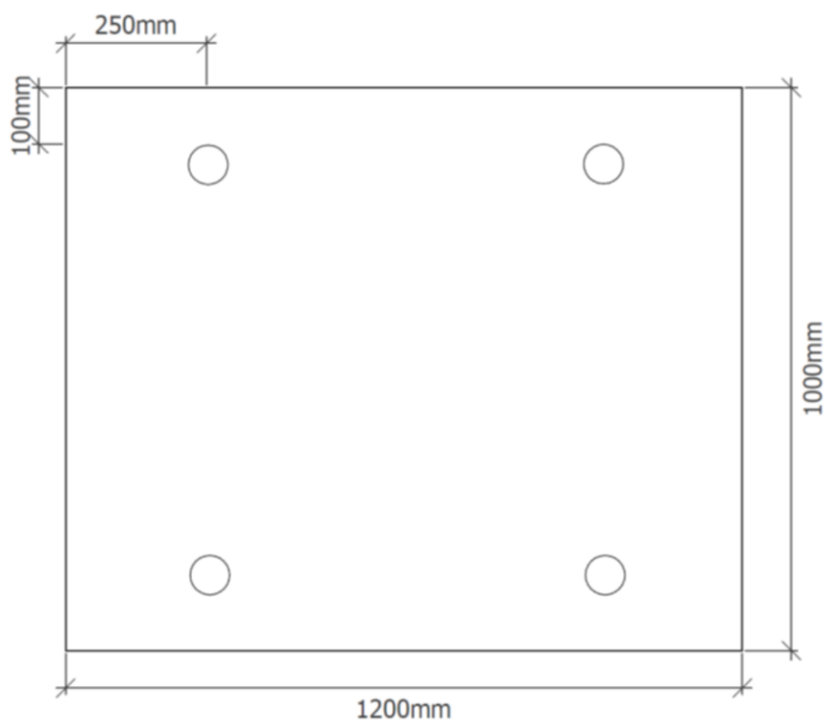
Figure 4.b – Fixations mécaniques préalables des panneaux de 1 200 mm × 600 mm ou 1 200 mm × 1 000 mm
