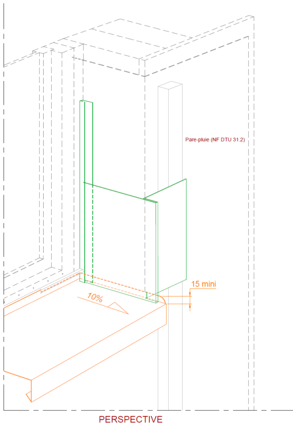
Figure 17 – Pose sur COB/CLT – perspective sur habillage de baie - menuiserie en tunnel intérieur - hauteurs de pose \leq 18 m pour les situations a, b et c et < 10 m en situation d
