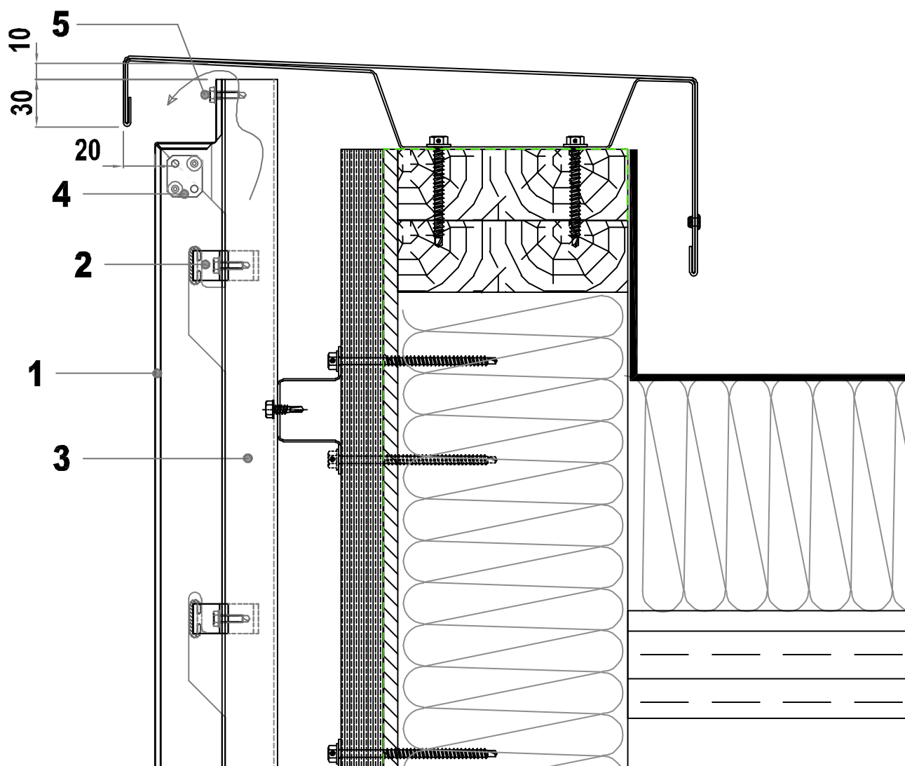
Figure 11 – Pose sur COB/CLT - Acrotère - coupe verticale
