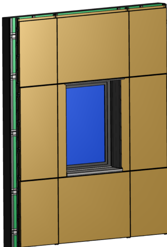
Etape 8 – Pose de l'habillage de linteau
