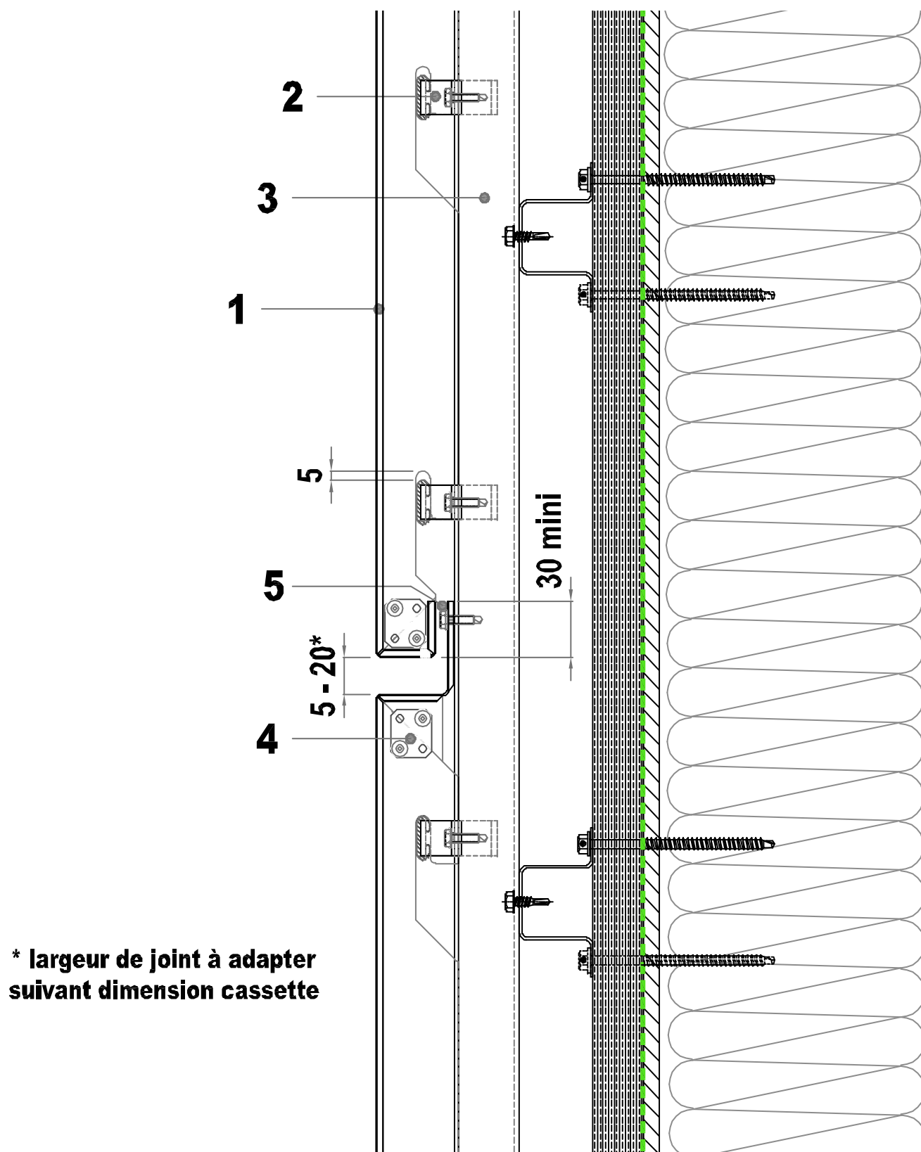
Figure 8a – Pose sur COB/CLT - Joint horizontal - coupe verticale - lisse horizontale métal
