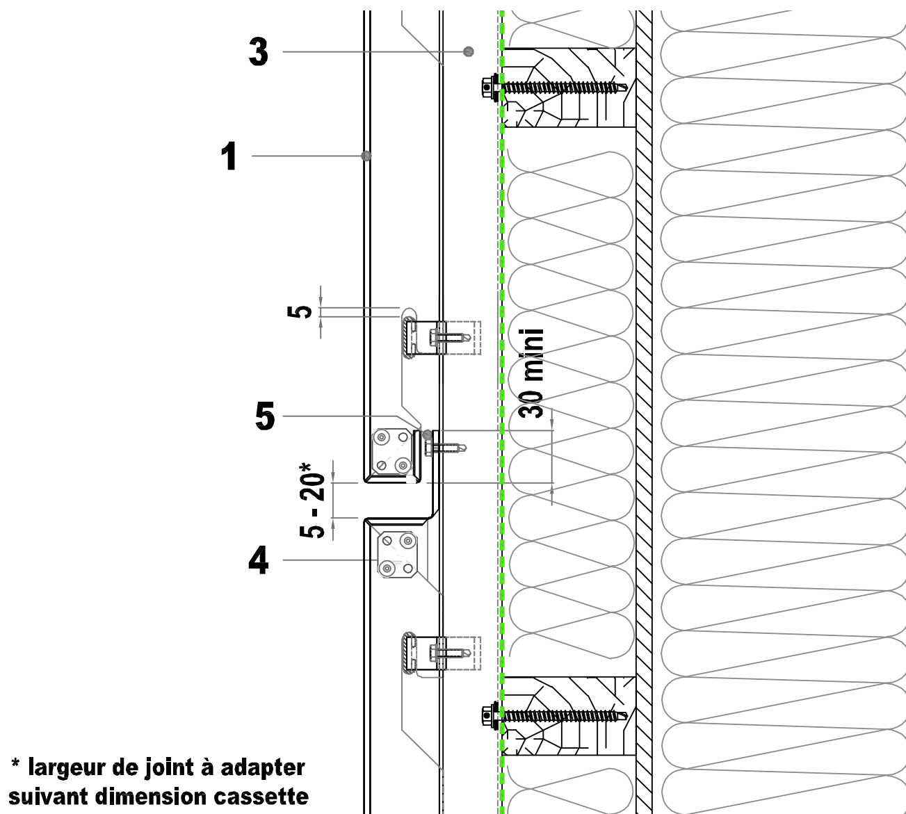
Figure 8d - Pose sur COB/CLT - Joint horizontal - coupe verticale - isolation thermique par l'extérieur
