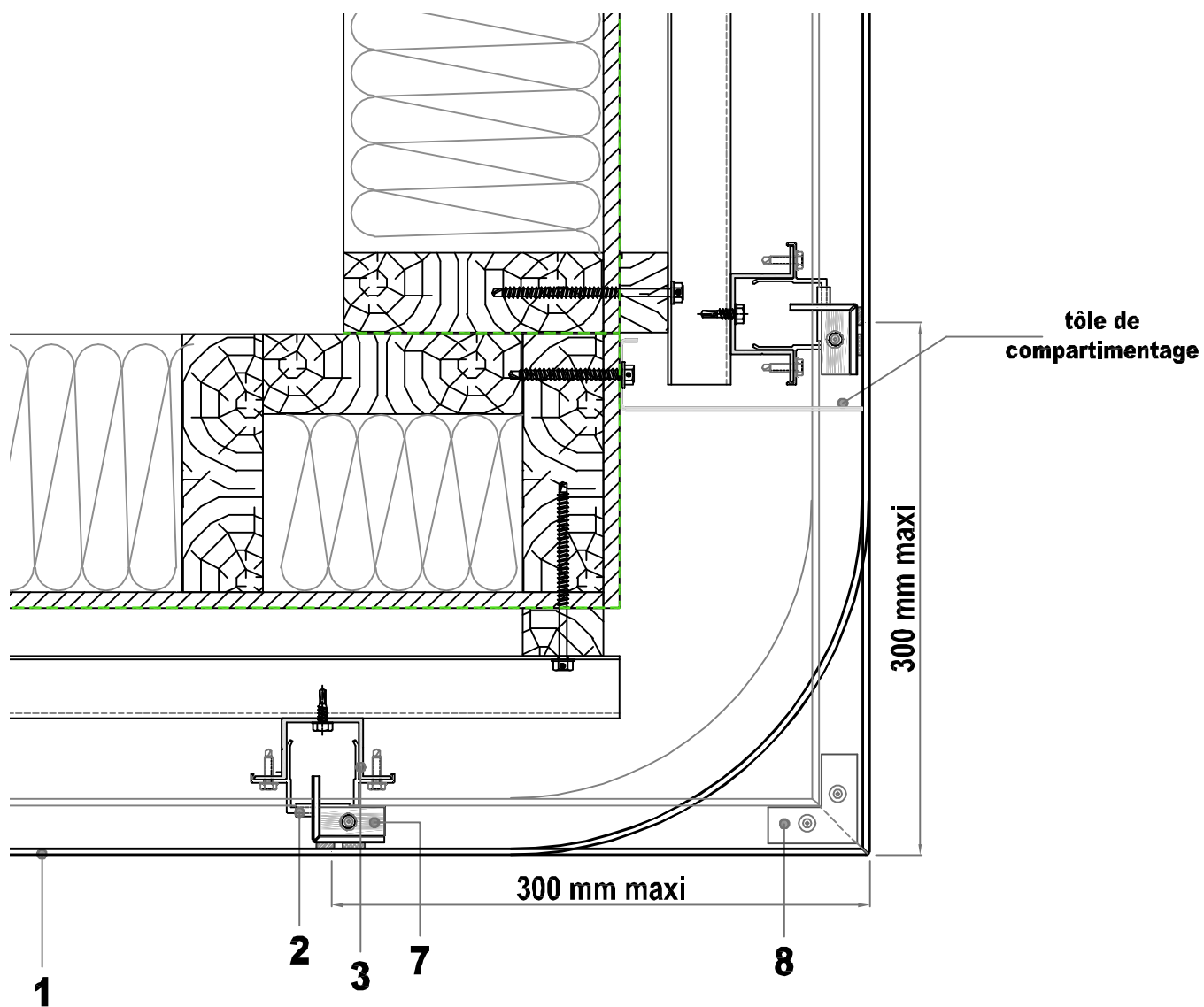
Figure 12b – Pose sur COB/CLT - Angle sortant - coupe horizontale
