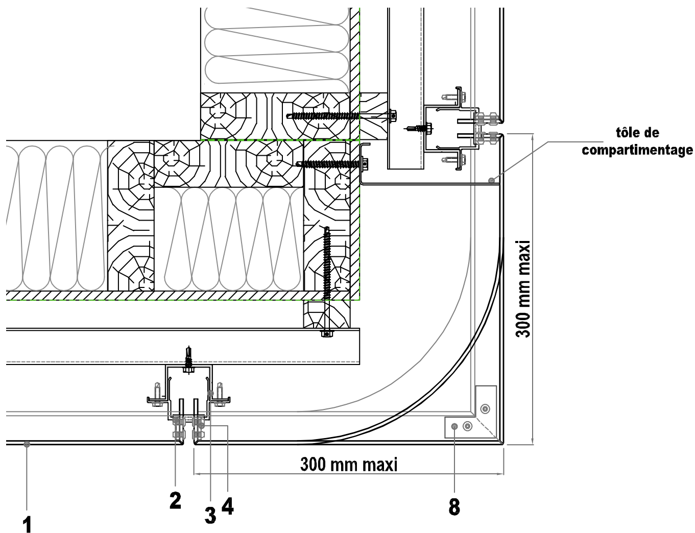
Figure 12a – Pose sur COB/CLT – Angle sortant - coupe horizontale
