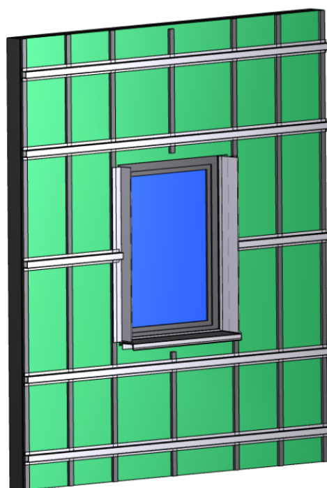
Etape 4 – Pose des traverses horizontales.
