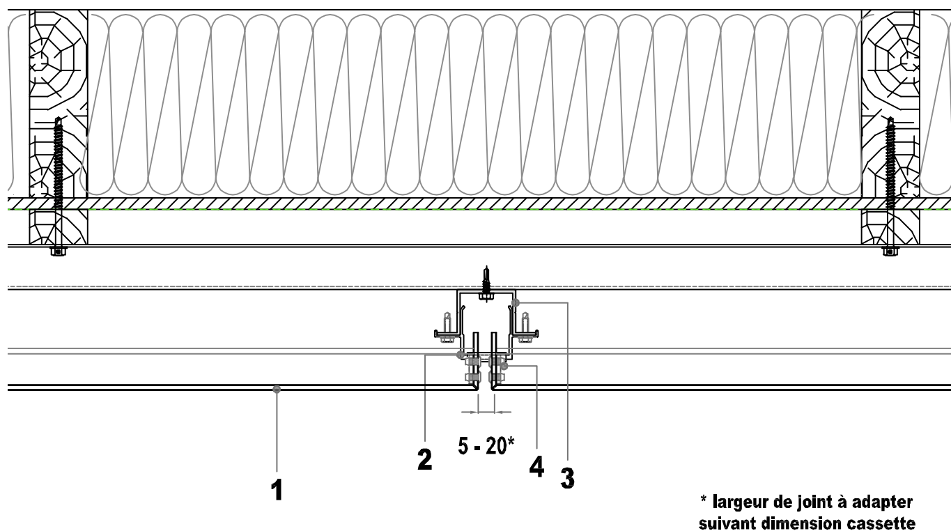
Figure 9a – Pose sur COB/CLT - Joint vertical - coupe horizontale – lisse horizontale métal
