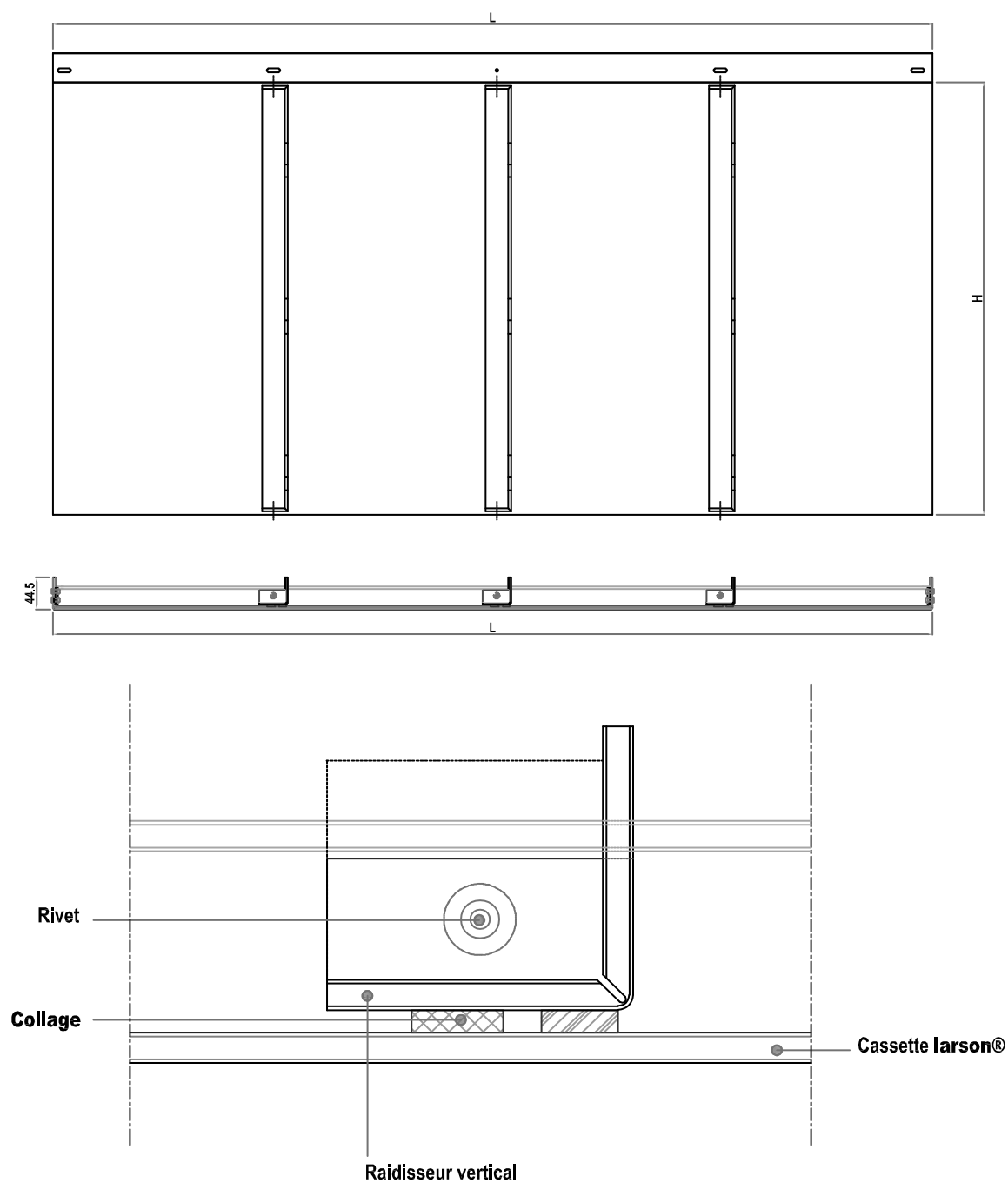
Figure 3a – Raidisseur vertical collé
