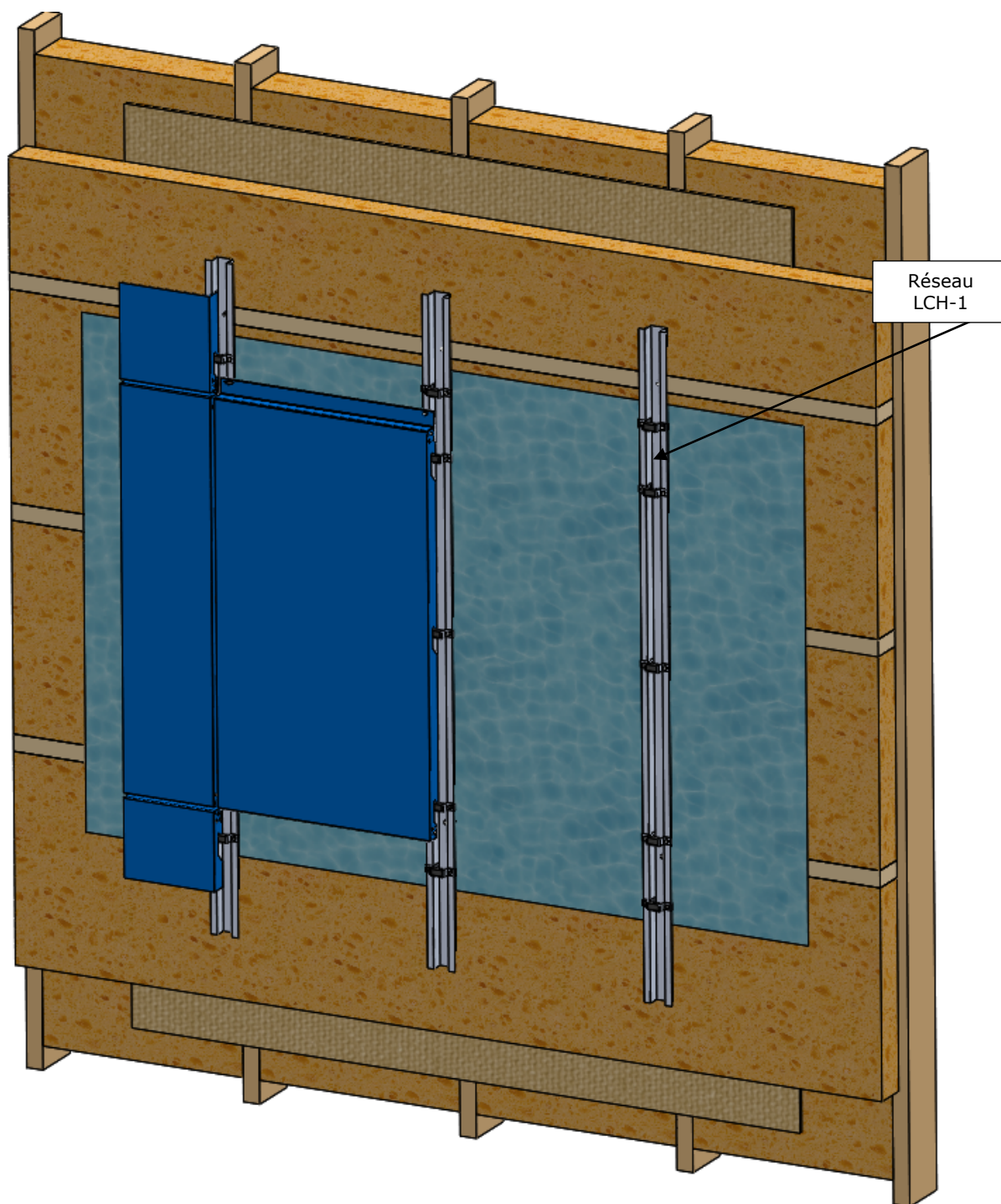
Figure 1c – Principe de mis en œuvre du système LARSON cassette sur COB/CLT avec complément d'isolation
