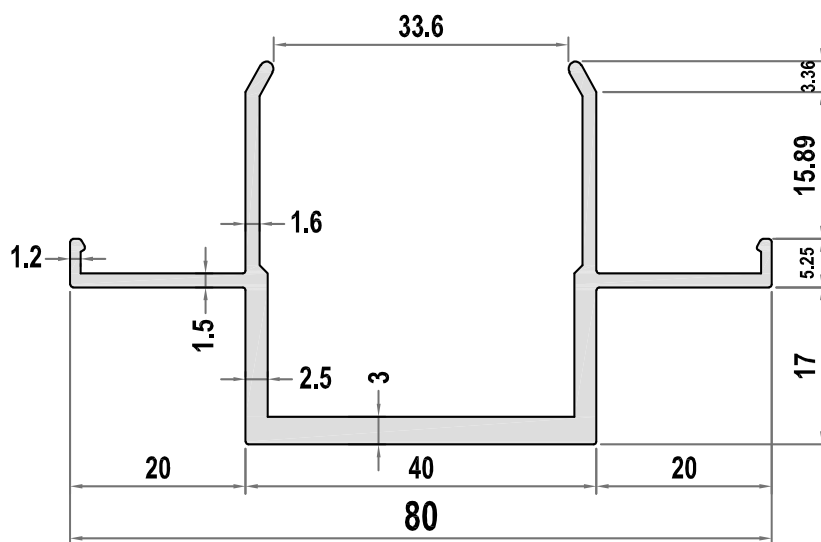
Figure 5b – Description de la pièce de suspension LC-3
