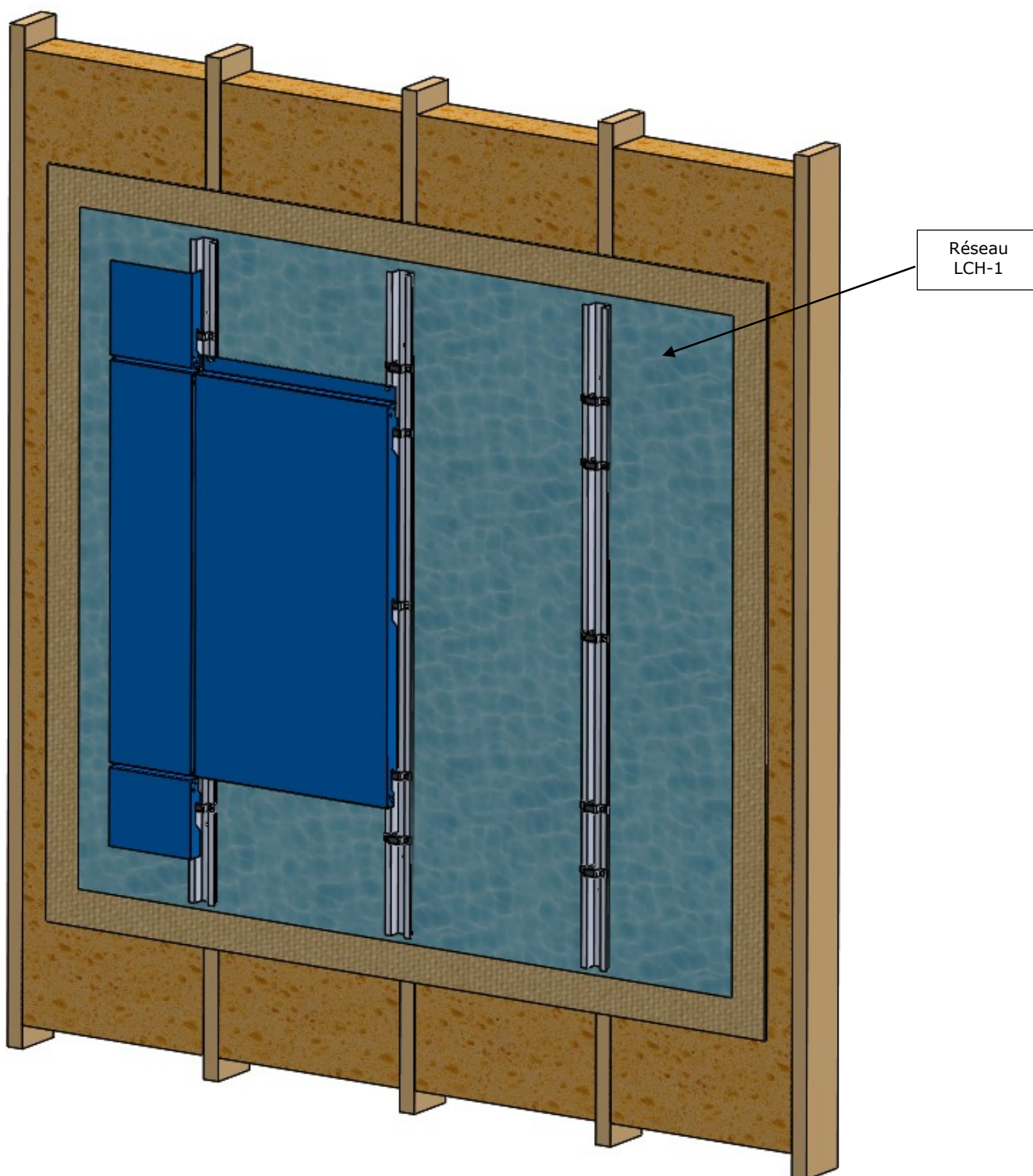
Figure 1b – Principe de mise en œuvre du système LARSON cassette sur COB/CLT en simple réseau
