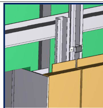
Etape 6 – Pose des cassettes larson® en allège.
