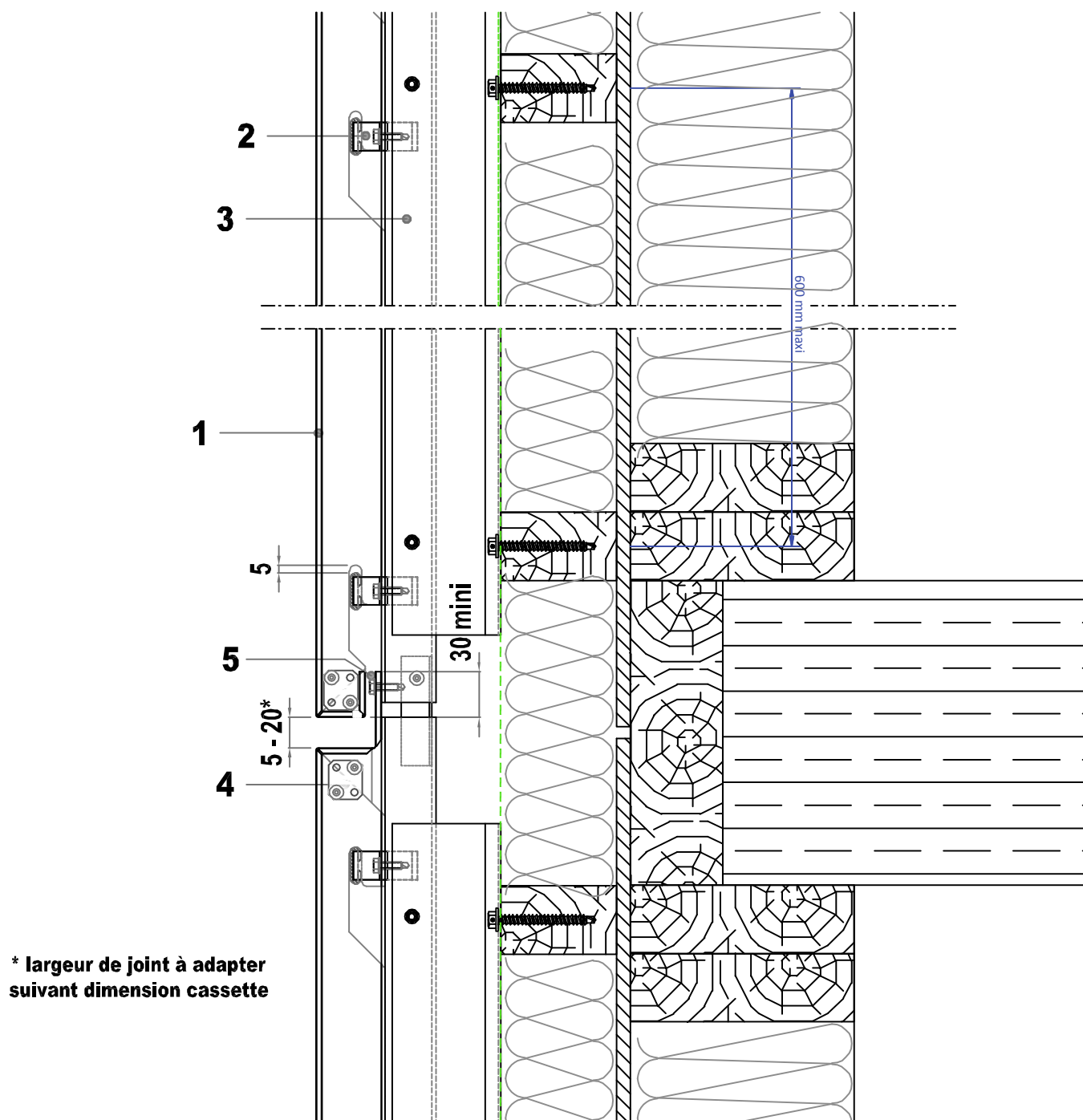
Figure A2 – Fractionnement de l'ossature au droit de chaque plancher
