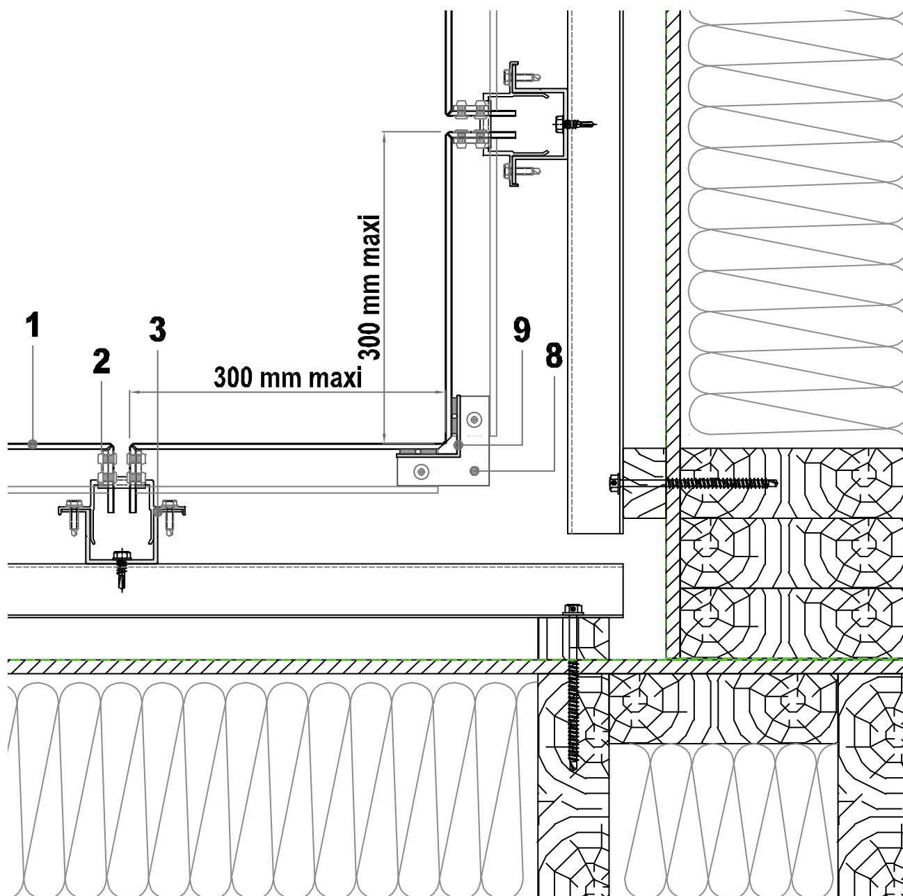
Figure 13a – Pose sur COB/CLT – Angle rentrant - coupe horizontale
