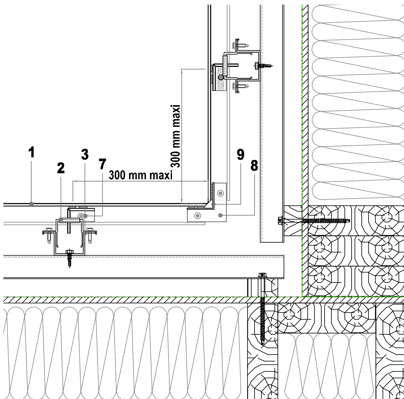
Figure 13b – Pose sur COB/CLT - Angle rentrant - coupe horizontale
