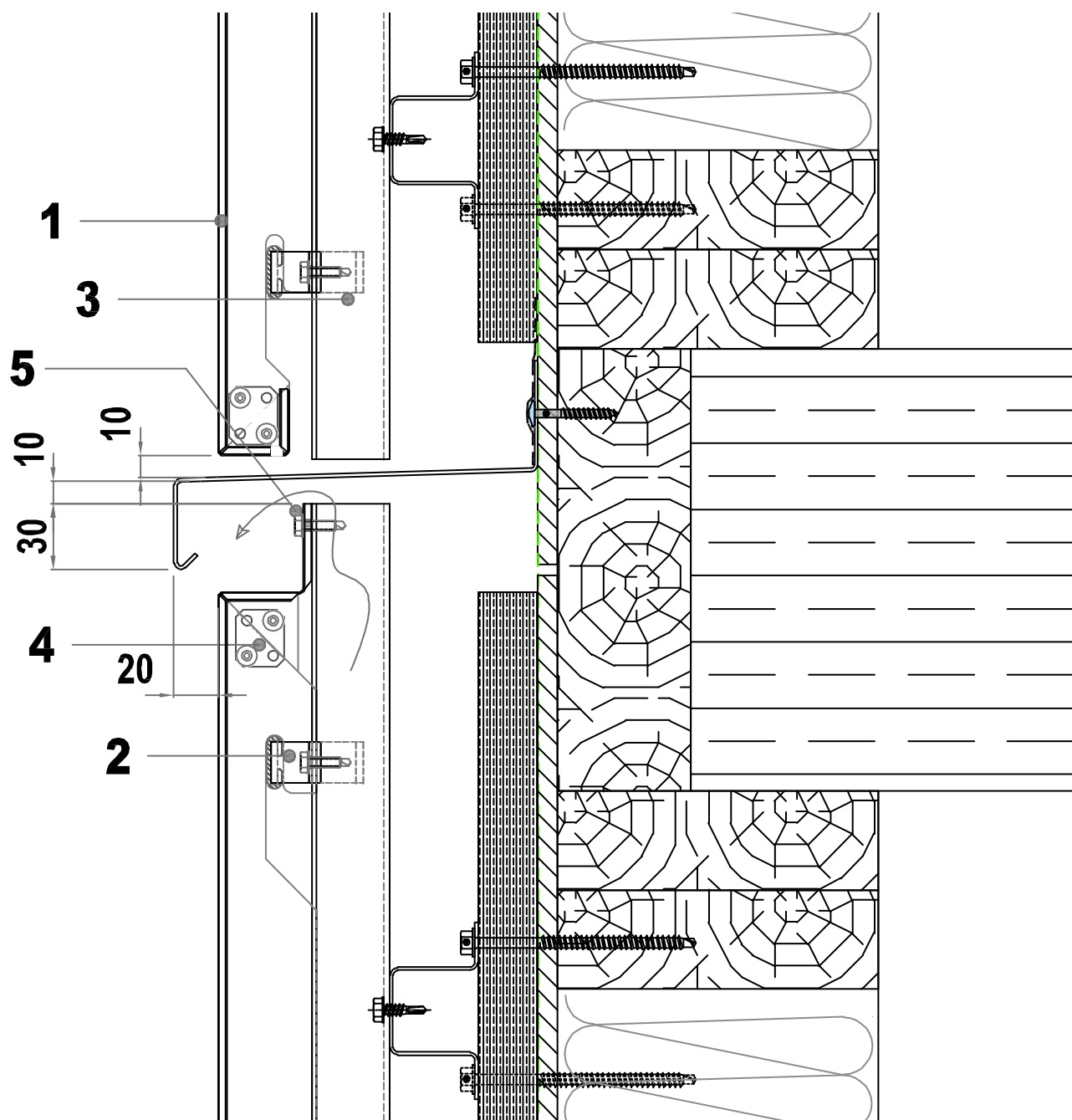
Figure 10b – Pose sur COB/CLT - Fractionnement de la lame d'air – coupe verticale
