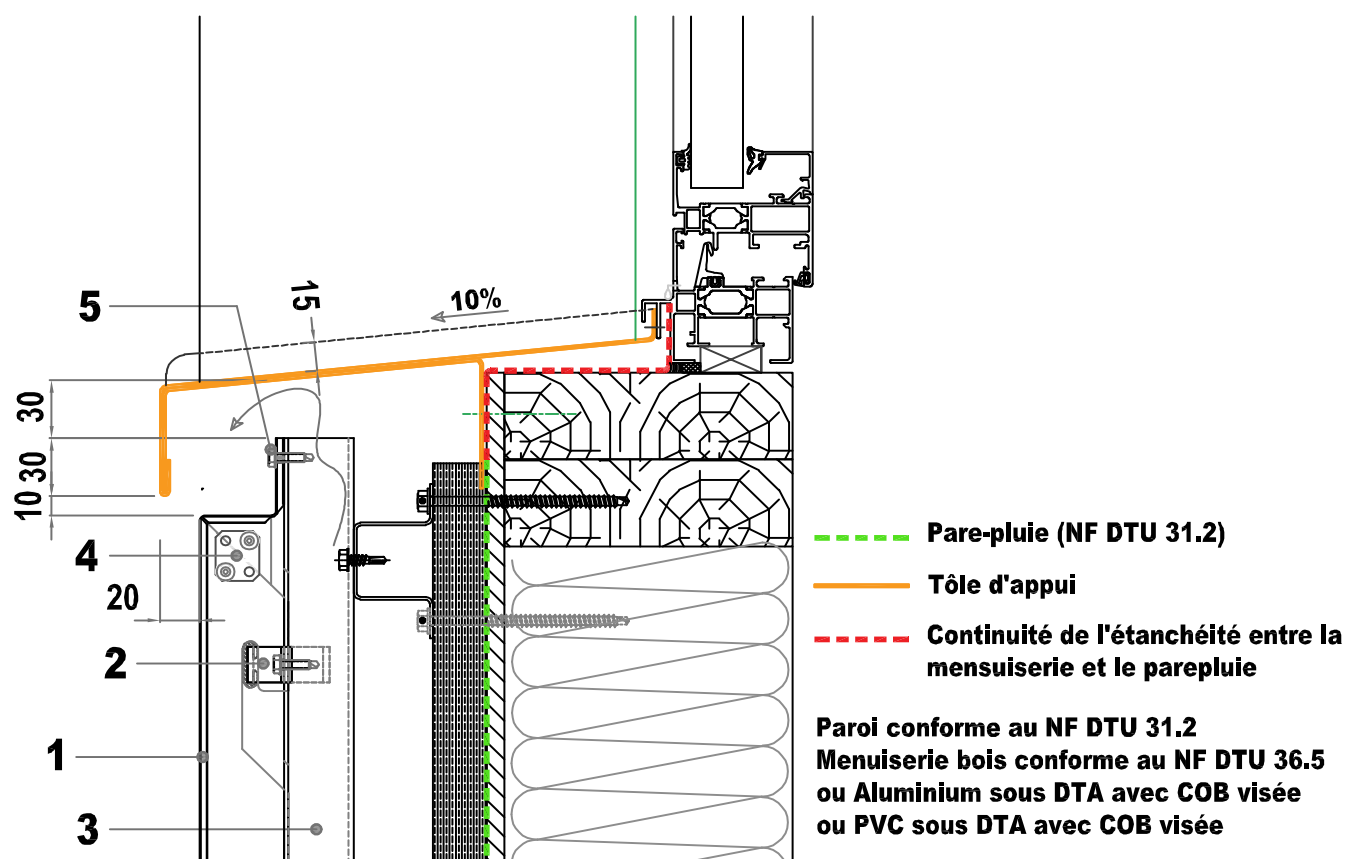
Figure 15 – Pose sur COB/CLT – appui de baie – coupe verticale - menuiserie en tunnel intérieur - hauteurs de pose \leq 18 m pour les situations a, b et c et < 10 m en situation d
