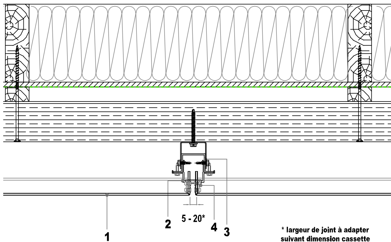
Figure 9b bis – Pose sur COB/CLT - Joint vertical - coupe horizontale – lisse horizontale bois avec profil U de réglage
