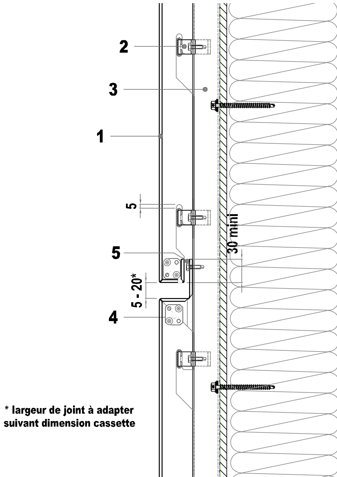
Figure 8c - Pose sur COB/CLT - Joint horizontal - coupe verticale - ossature de bardage simple réseau
