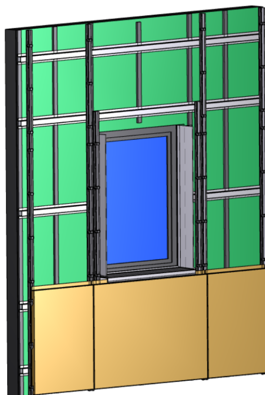
Etape 6 – Pose des cassettes larson® en allège.
