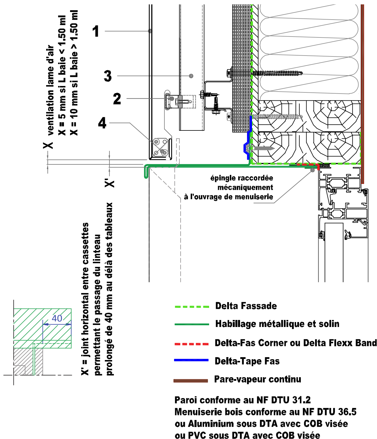
Figure 22 – Pose sur COB/CLT – Linteau de baie – coupe verticale - menuiserie en tunnel intérieur et membrane de protection à l'eau sous Avis Technique (ex : Doerken Delta Fassade Plus) - hauteurs de pose ≤ 28 m pour les situations a, b et c et < 18 m en situation d
