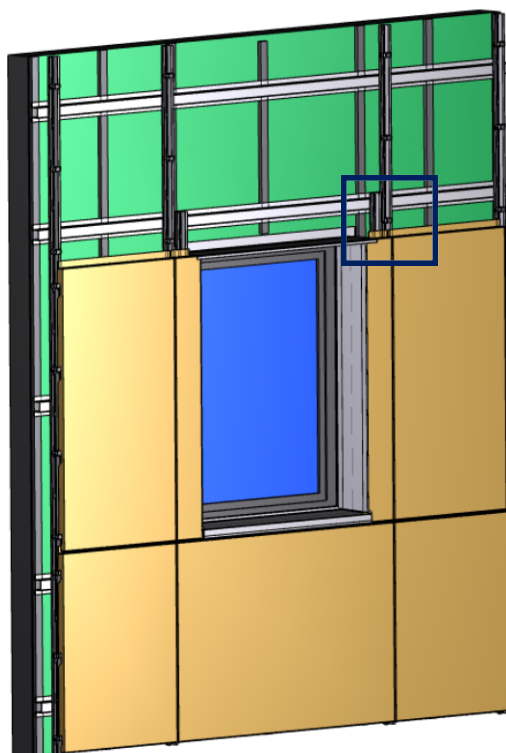
Etape 8 – Pose de l'habillage de linteau
