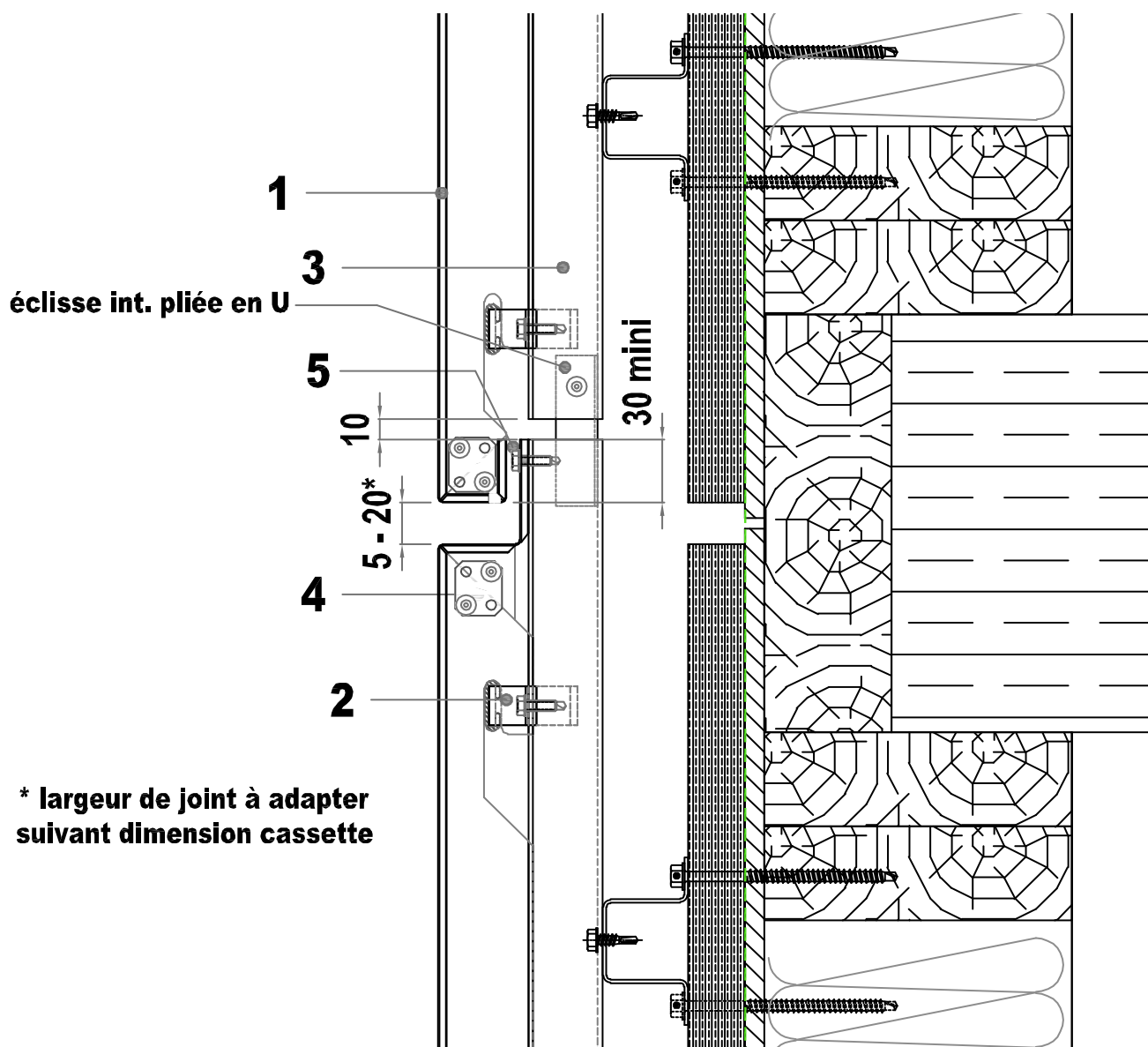
Figure 10a – Pose sur COB/CLT - Fractionnement de l'ossature au droit de chaque plancher – coupe verticale
