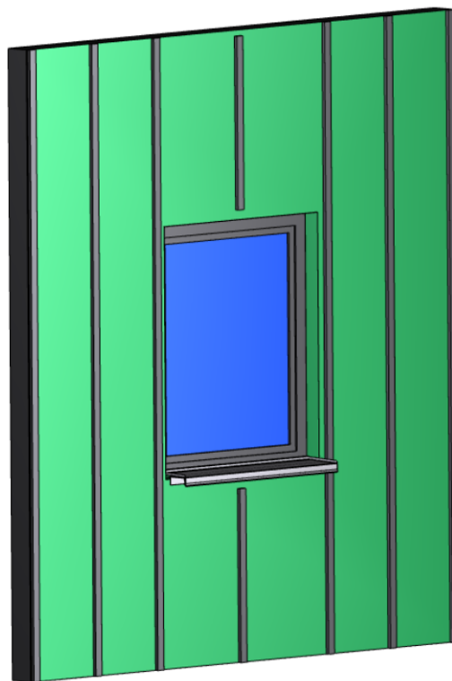
Etape 2 – Pose du support de bavette et de la bavette à oreilles.
