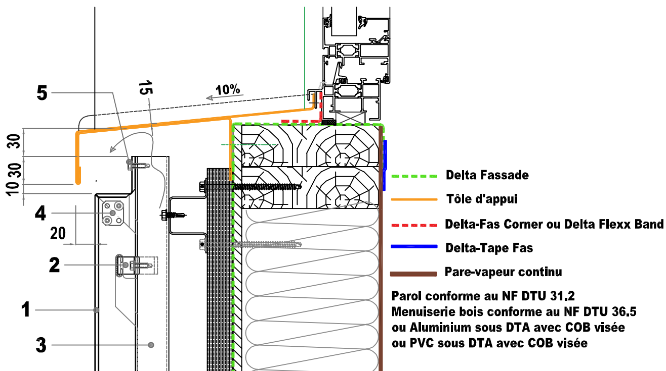
Figure 23 – Pose sur COB/CLT – appui de baie – coupe verticale - menuiserie en tunnel intérieur et membrane de protection à l'eau sous Avis Technique (ex : Doerken Delta Fassade Plus)- hauteurs de pose \leq 28 m pour les situations a, b et c et < 18 m en situation d
