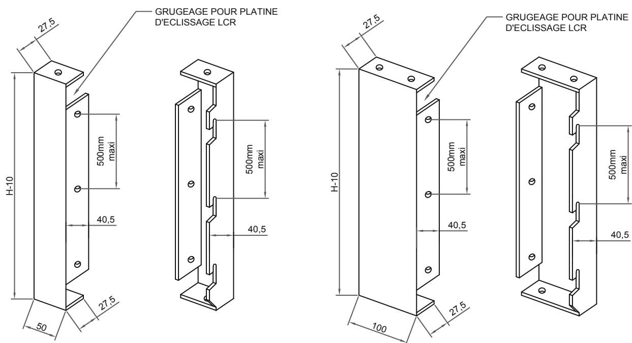
Figure 3b – Fixation déportée rivetée (pour tableau ou JD sismique)
