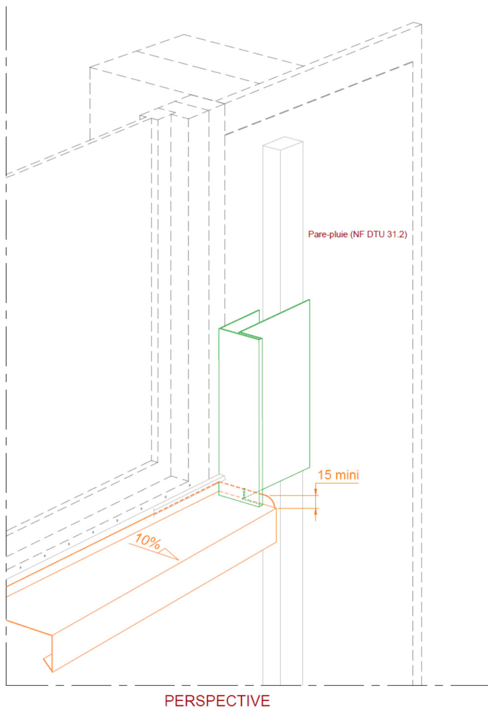
Figure 21 – Pose sur COB/CLT – perspective sur habillage de baie - menuiserie en tunnel extérieur - hauteurs de pose \leq 18 m pour les situations a, b et c et < 10 m en situation d
