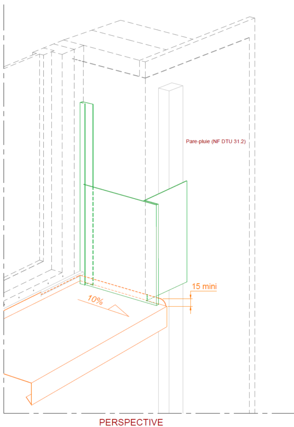
Figure 25 – Pose sur COB/CLT – perspective sur habillage de baie - menuiserie en tunnel intérieur et membrane de protection à l'eau sous Avis Technique (ex : Doerken Delta Fassade Plus) - hauteurs de pose \leq 28 m pour les situations a, b et c et < 18 m en situation d
