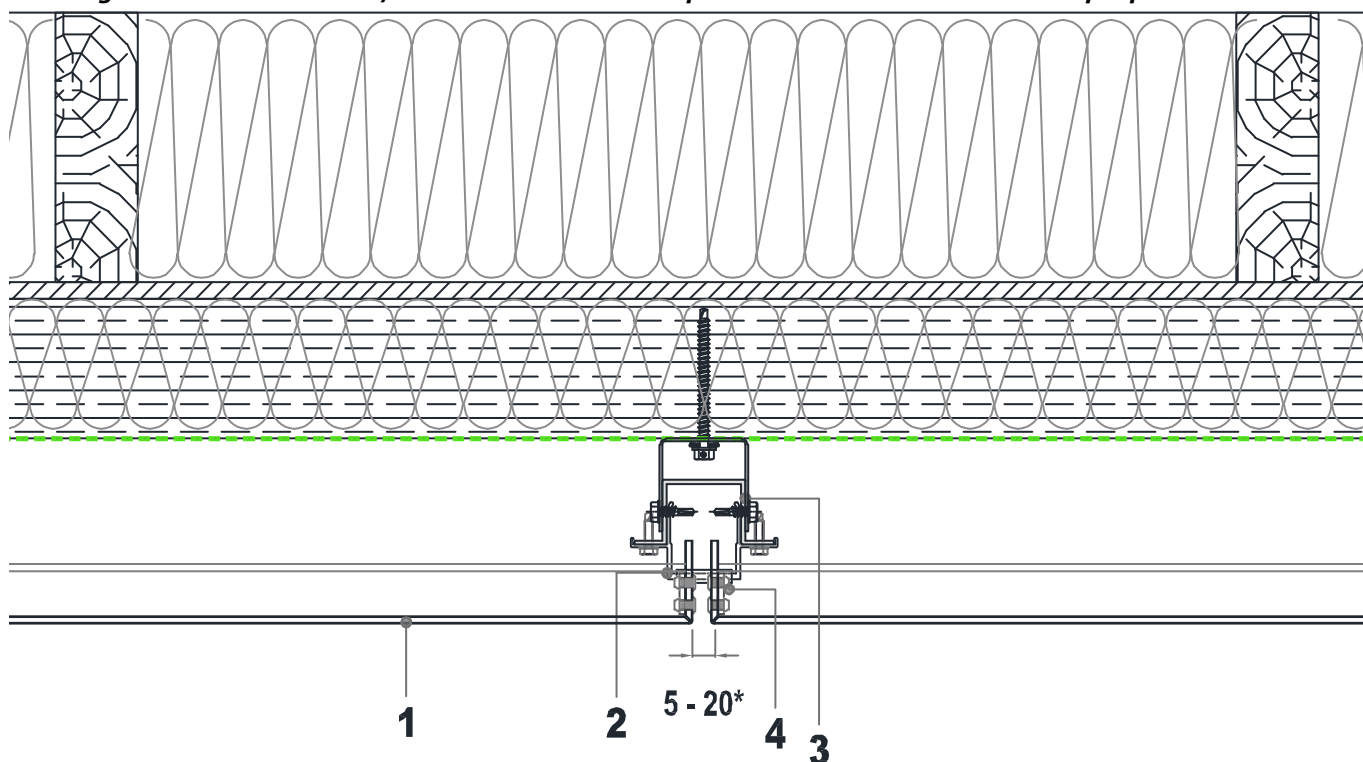
Figure 9d – Pose sur COB/CLT - Joint vertical - coupe horizontale – isolation thermique par l'extérieur
