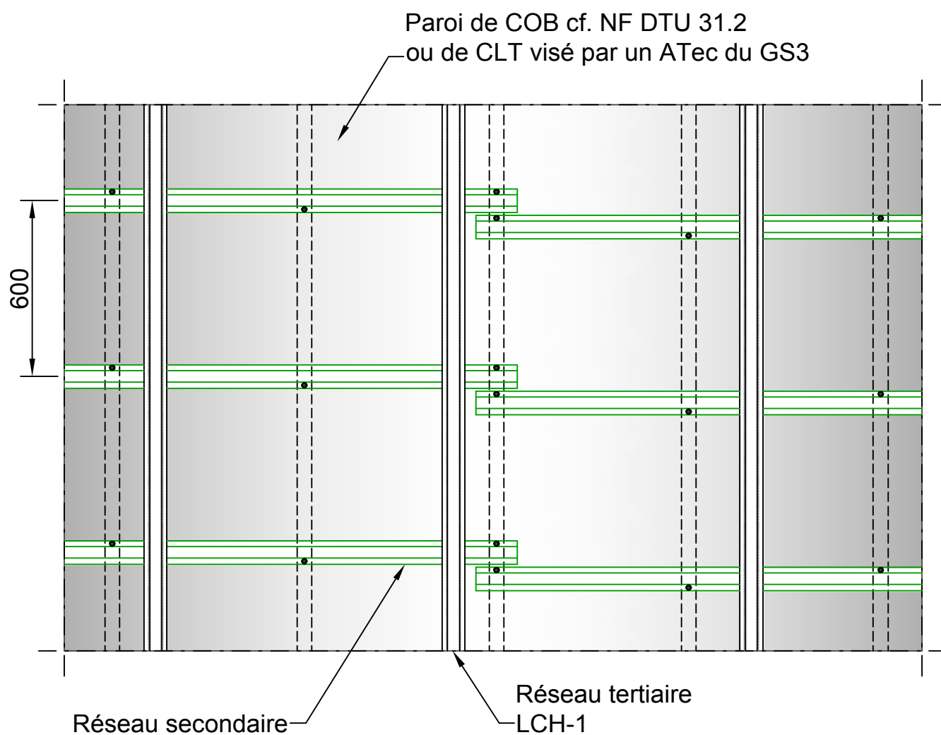
Figure 6 – Pose sur COB/CLT – Raccordement lisses horizontales secondaires et disposition de leurs fixations
