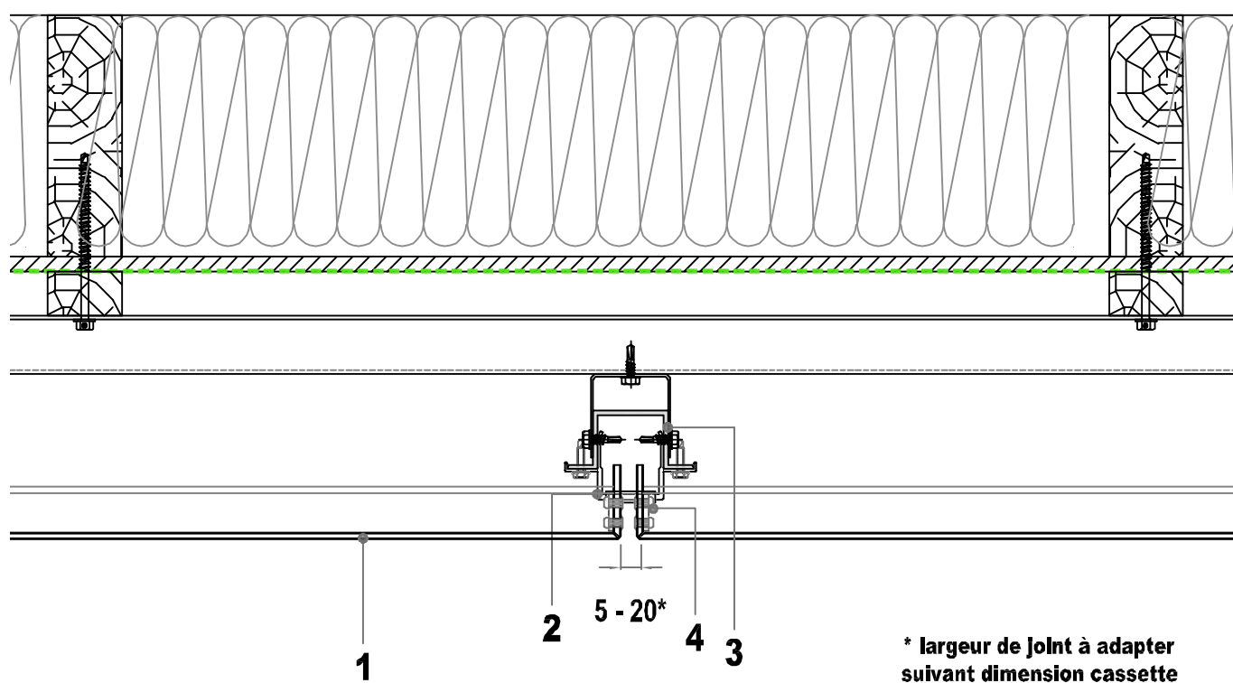
Figure 9a bis – Pose sur COB/CLT - Joint vertical - coupe horizontale – lisse horizontale métal avec profil U de réglage
