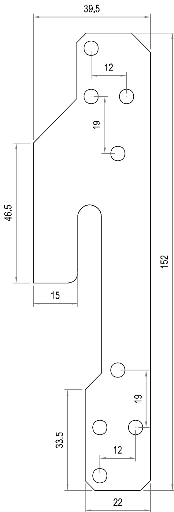
Figure 4b – LCR-45 – Renfort de d'encoche
