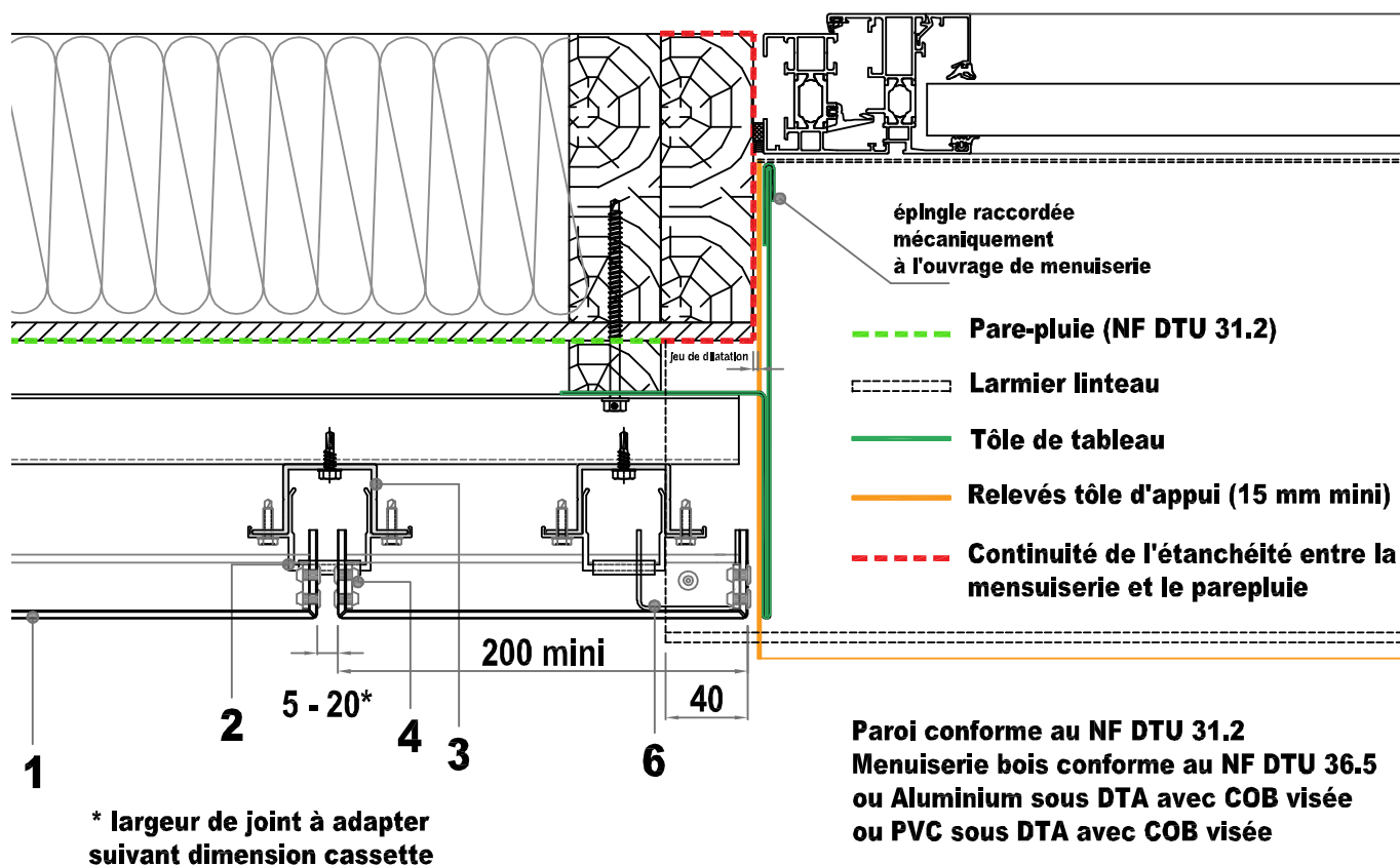
Figure 16 – Pose sur COB/CLT – tableau de baie – coupe horizontale - menuiserie en tunnel intérieur - hauteurs de pose \leq 18 m pour les situations a, b et c et < 10 m en situation d
