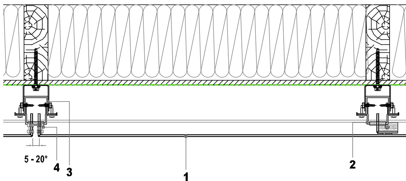
Figure 9c – Pose sur COB/CLT - Joint vertical - coupe horizontale – ossature de bardage simple réseau
