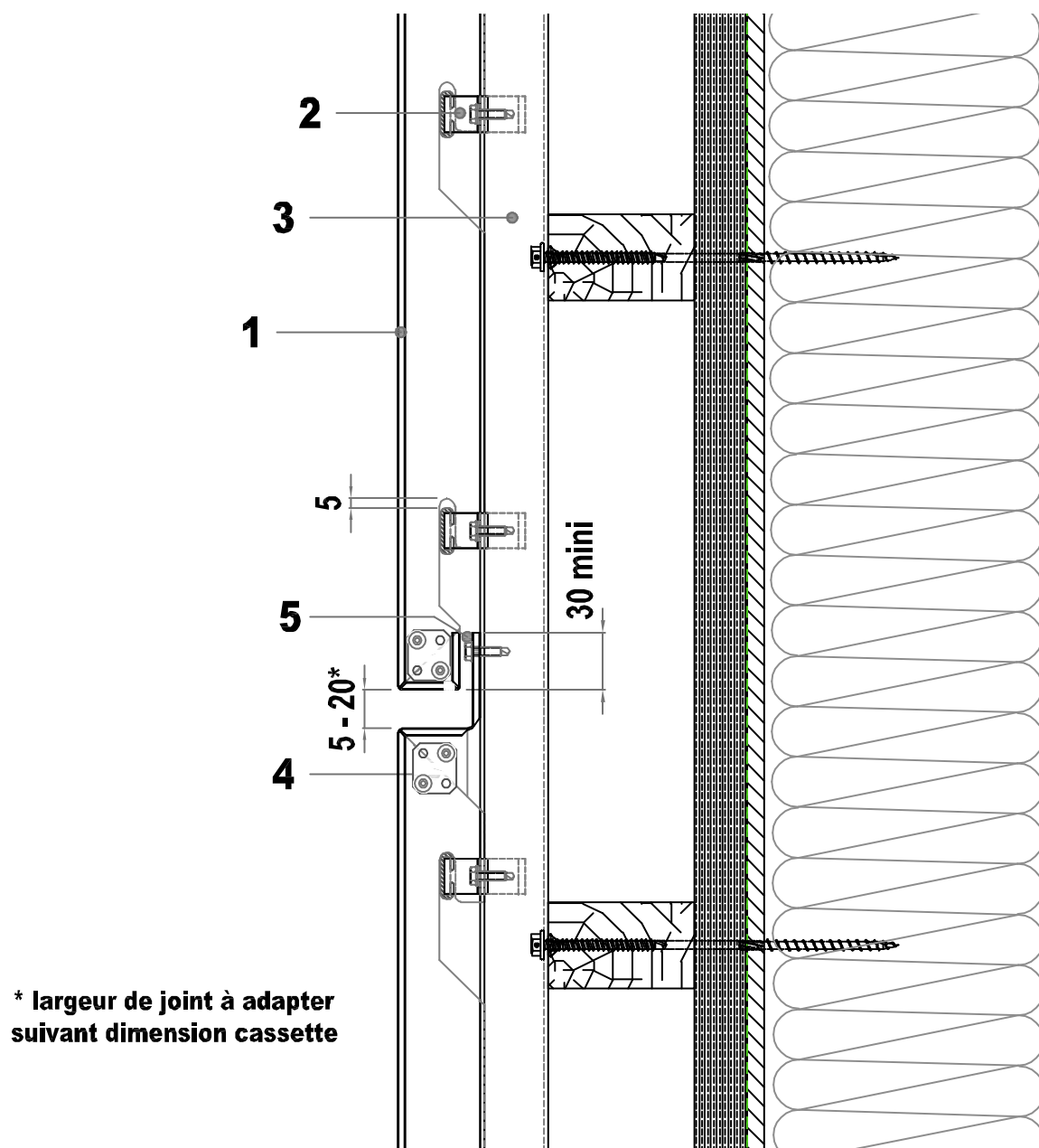
Figure 8b - Pose sur COB/CLT - Joint horizontal - coupe verticale - lisse horizontale bois
