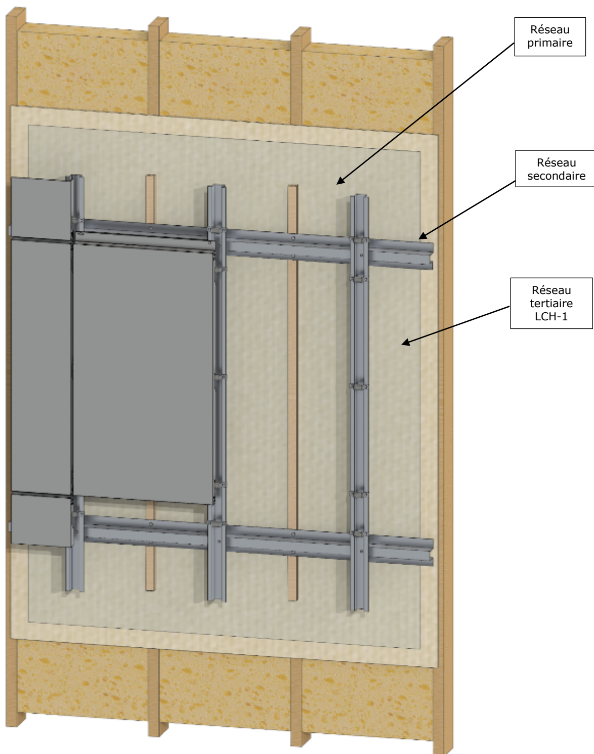
Figure 1a – Principe de mise en œuvre du système LARSON cassette sur COB/CLT en triple réseau
