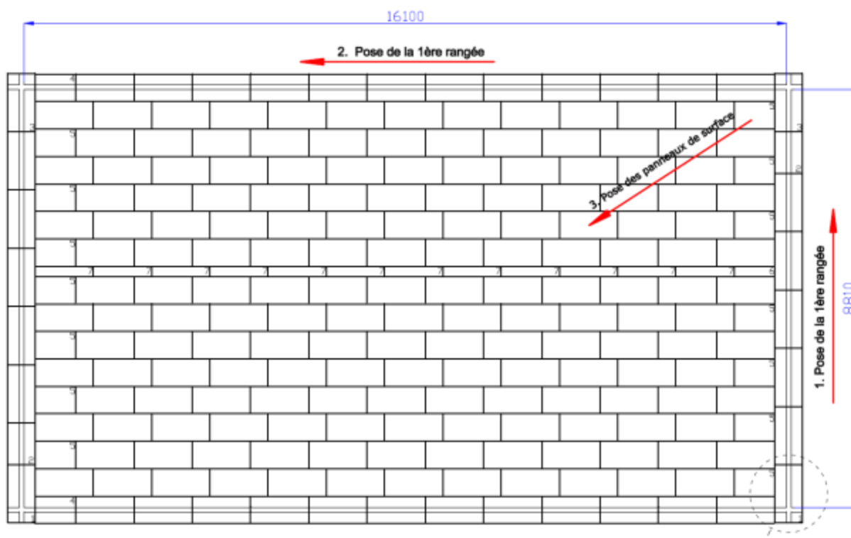
Figure 7 – Exemple de plan de pose
