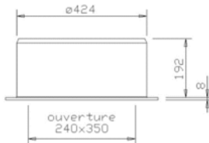
Figure 8b – Connecteur de rehausse DN/ID 425
