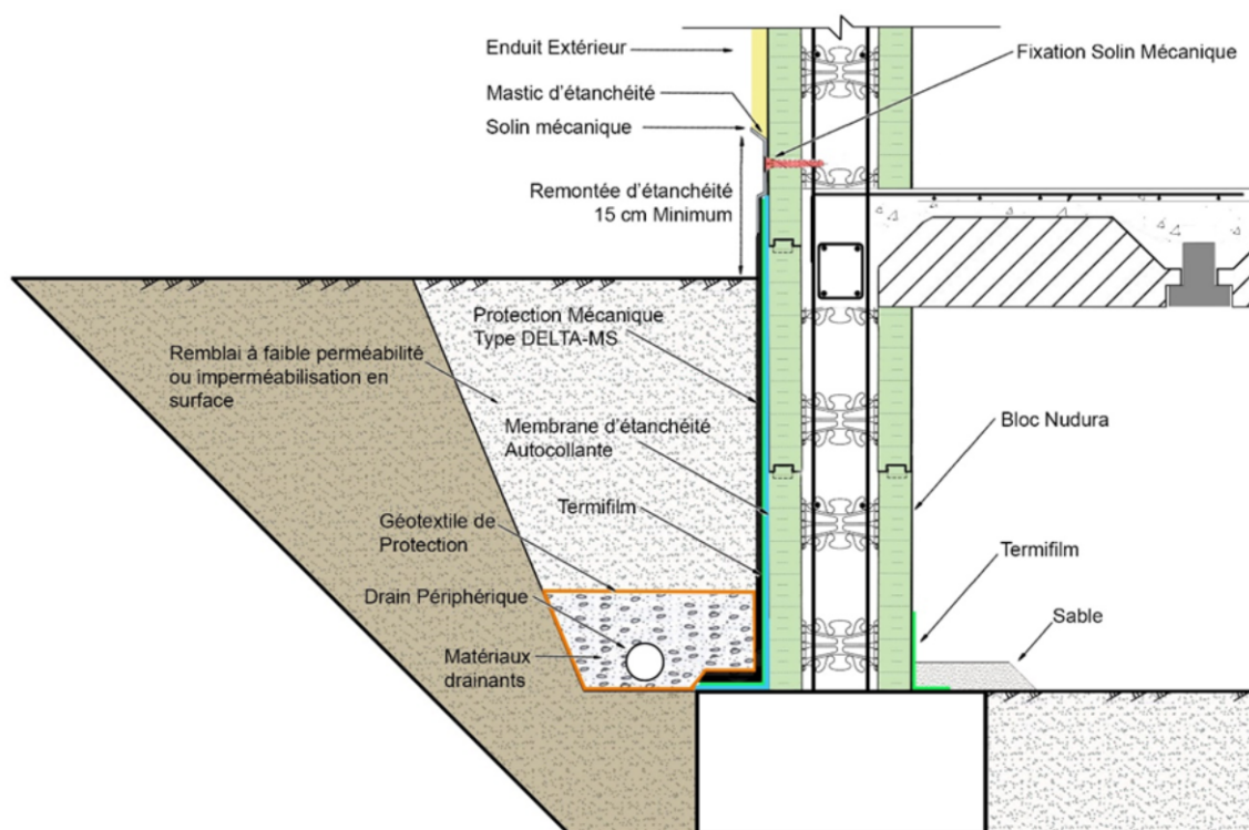
Figure 35 - Prévention contre les termites – Périphérie d'un vide sanitaire > 60 cm
