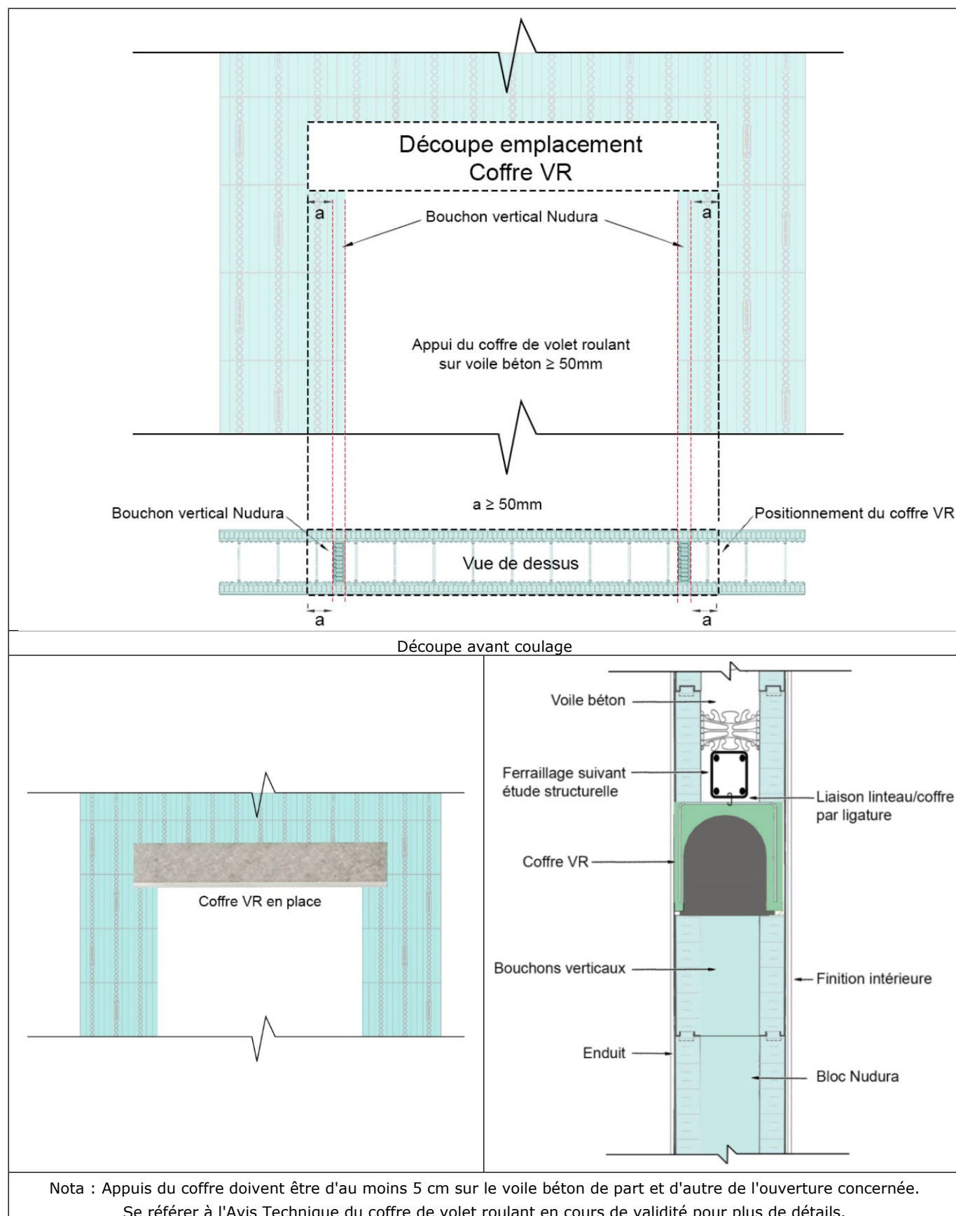
Figure 27 - Pose de coffres tunnels pour volets roulants
