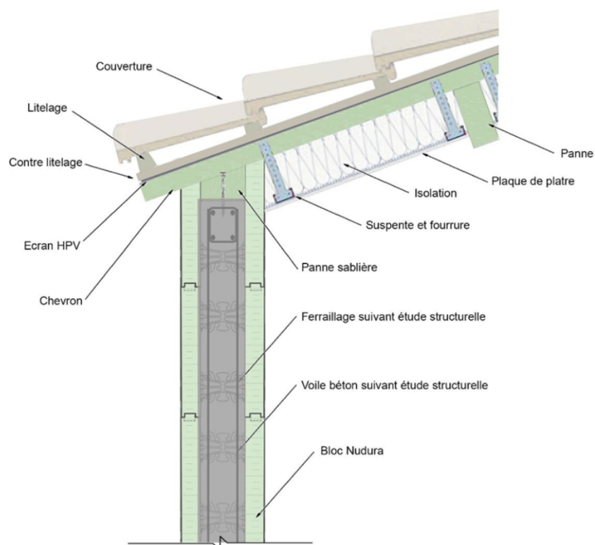
Figure 19 - Jonction Mur Nudura / Toiture (Charpente Traditionnelle)
