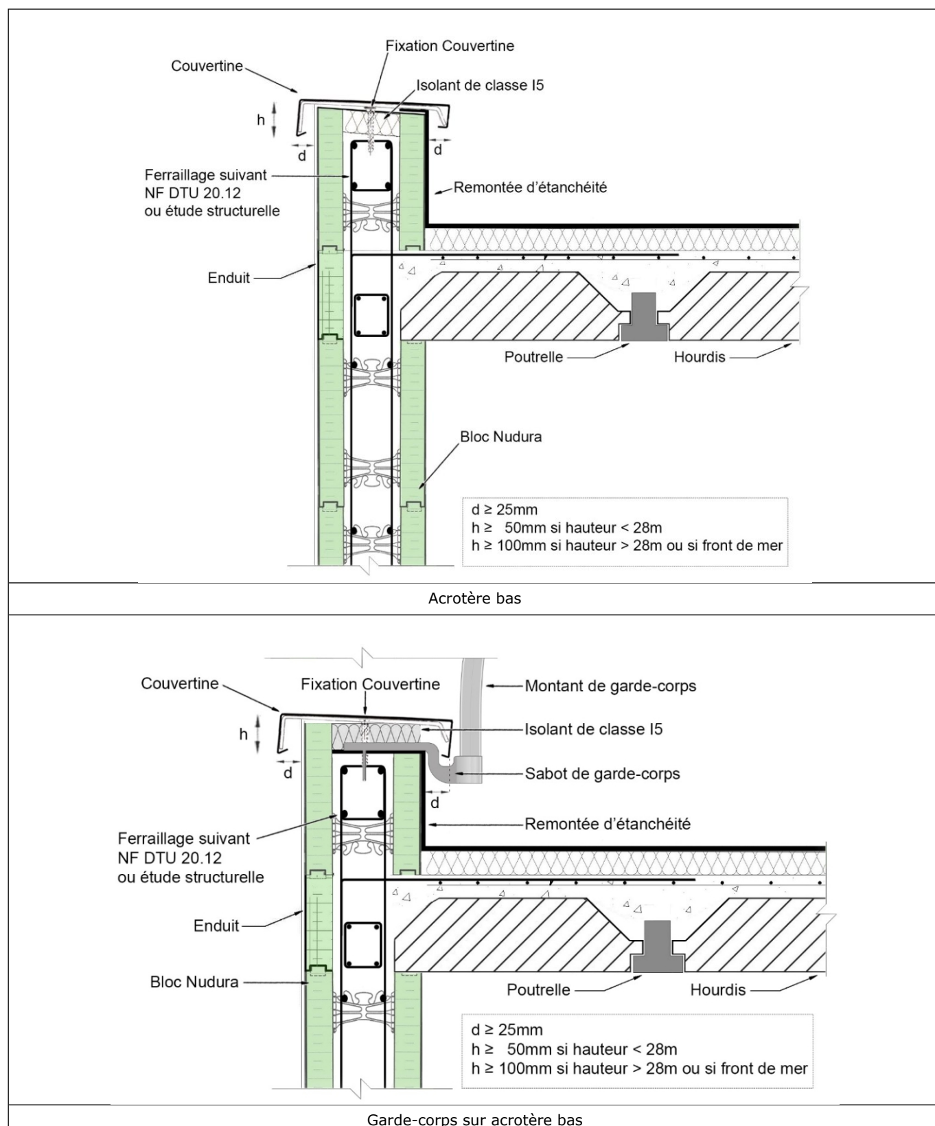
Figure 21 – Acrotères bas avec les blocs Nudura - voile béton d'épaisseur 152 mm ou 203 mm
