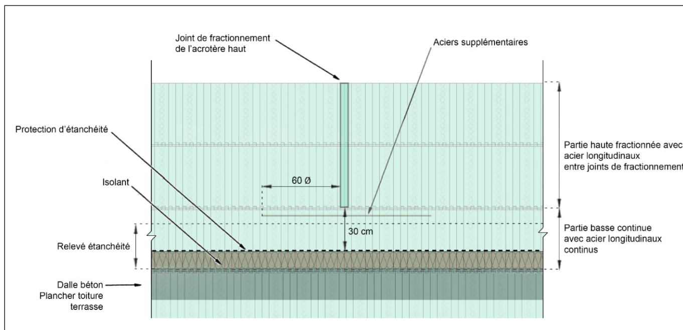
Joint de fractionnement acrotère haut
