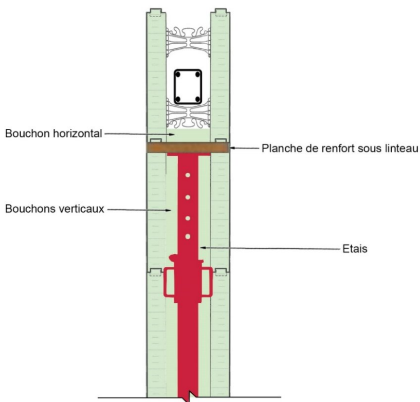
Figure 11 - Etalement des ouvertures avec les bouchons
