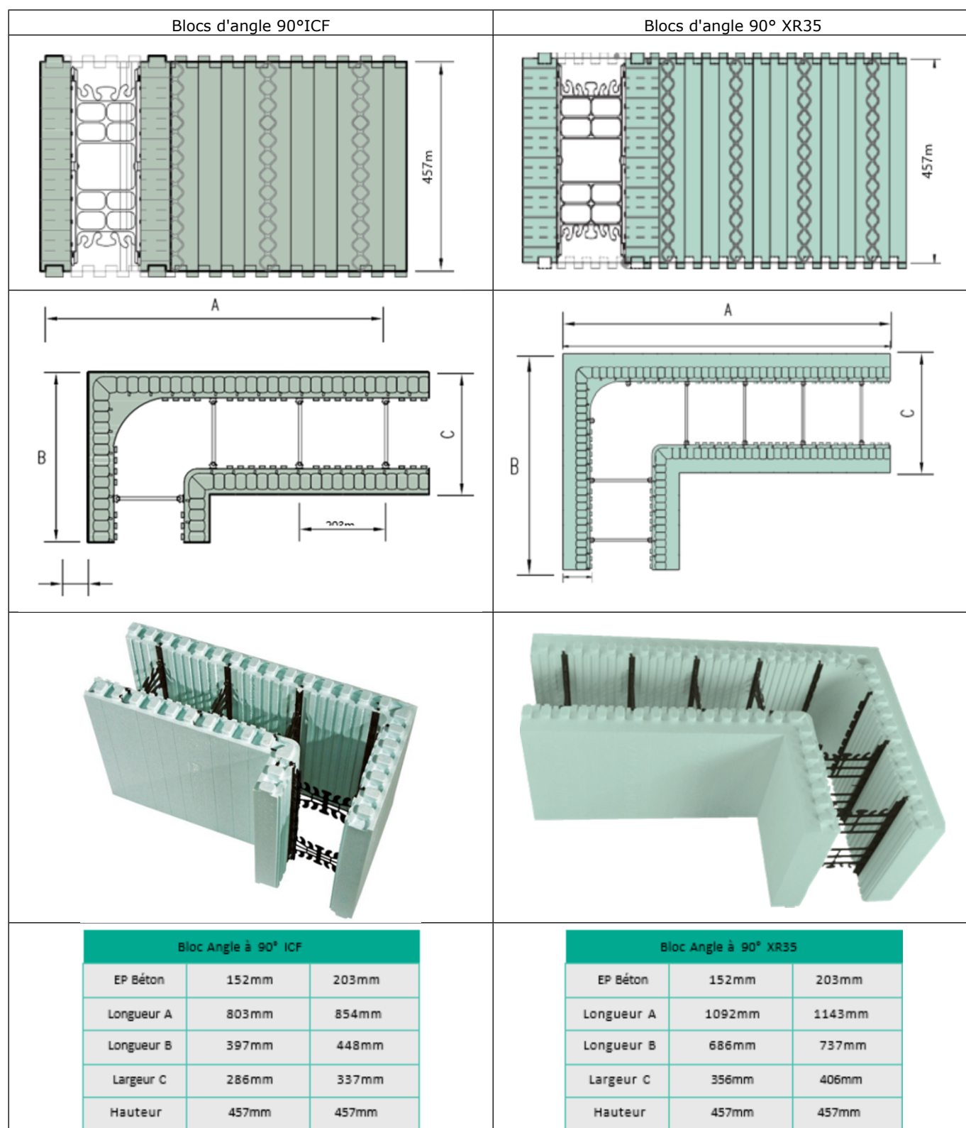
Figure 6 - Blocs d'angle 90° ICF et XR35
