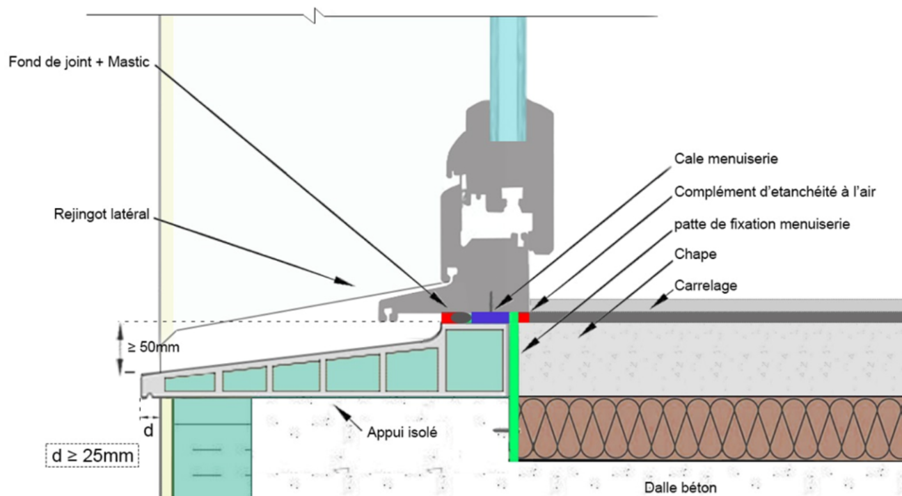
Figure 28 - Seuil classique
