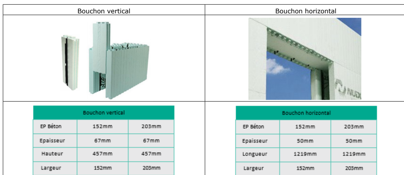
Figure 9 - Bouchon vertical et bouchon horizontal
