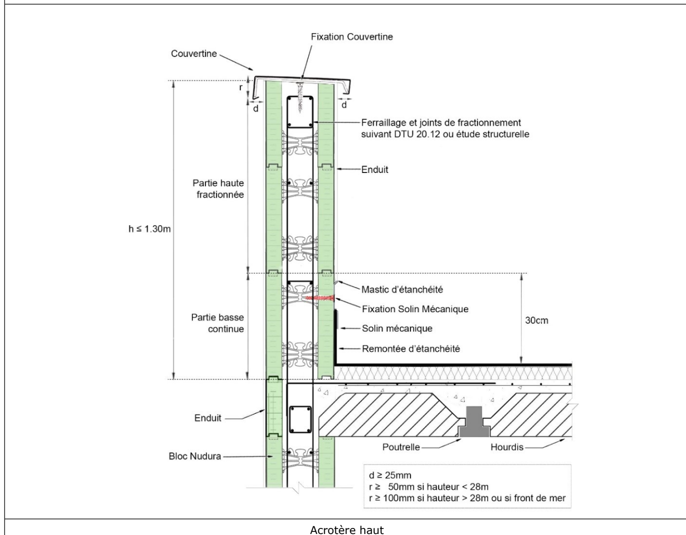
Figure 22 – Acrotères hauts avec les blocs Nudura - voile béton d'épaisseur 152 mm ou 203 mm
