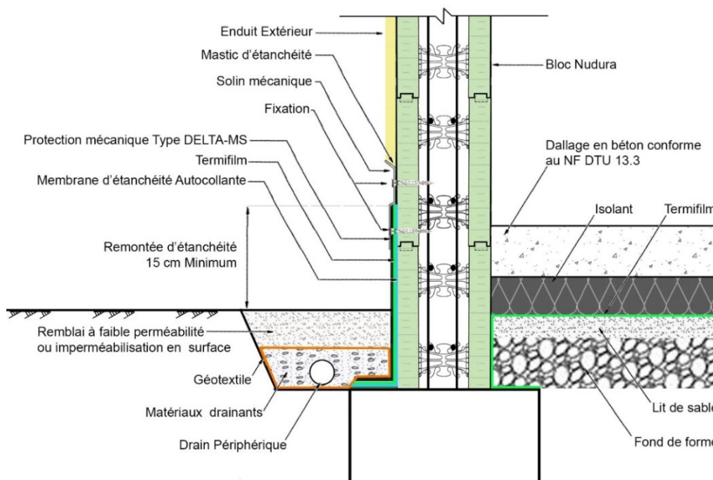
Figure 31 - Prévention contre les termites – Périphérie dallage sur terre-plein isolé et non porté
