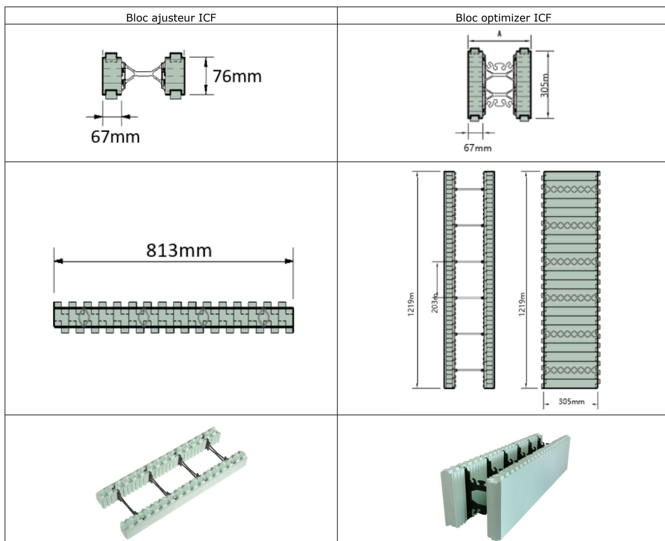
Figure 8 - Blocs ajusteur ICF et blocs Optimizer ICF
