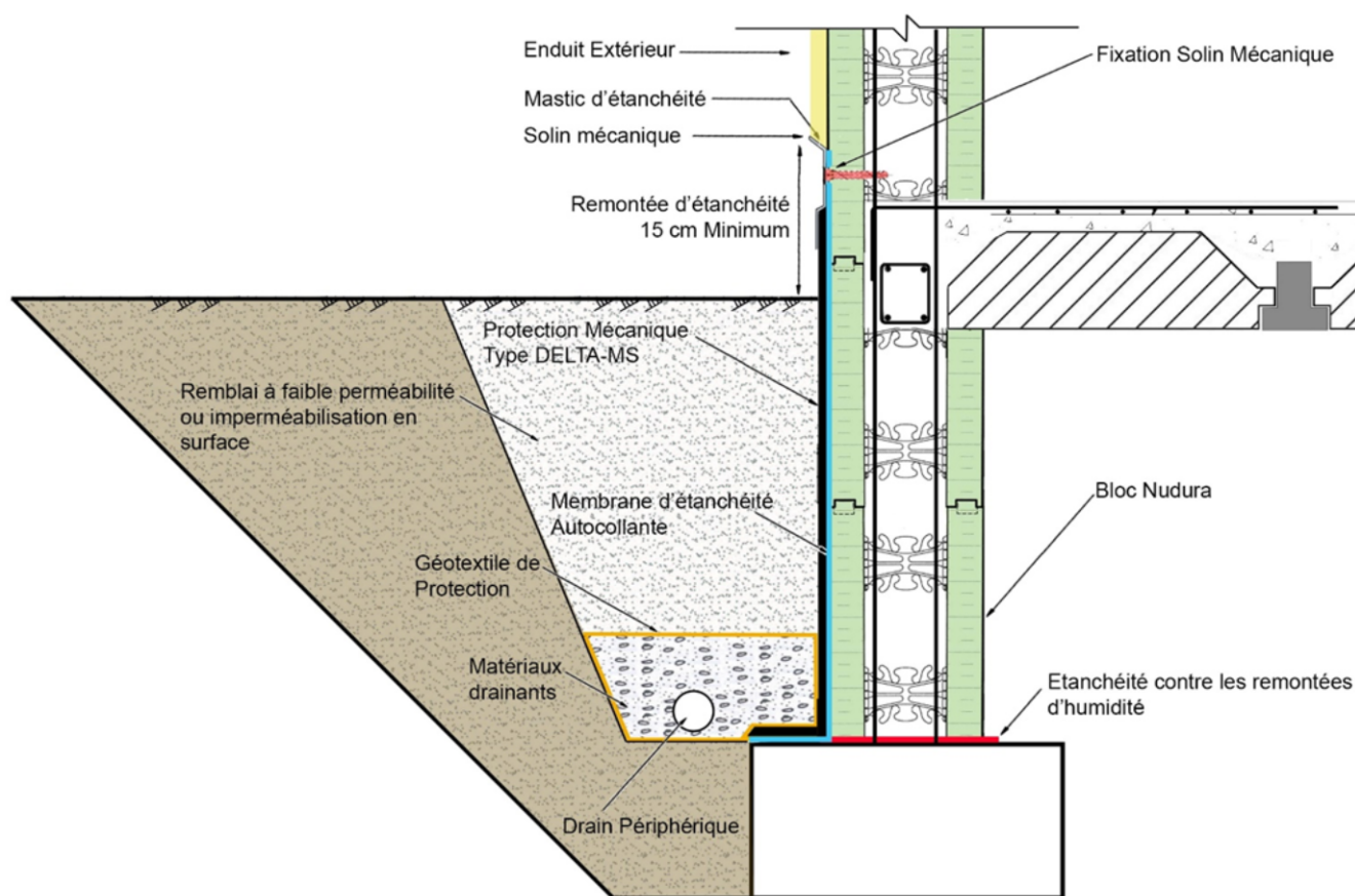
Figure 30 - Etanchéité des parois enterrées
