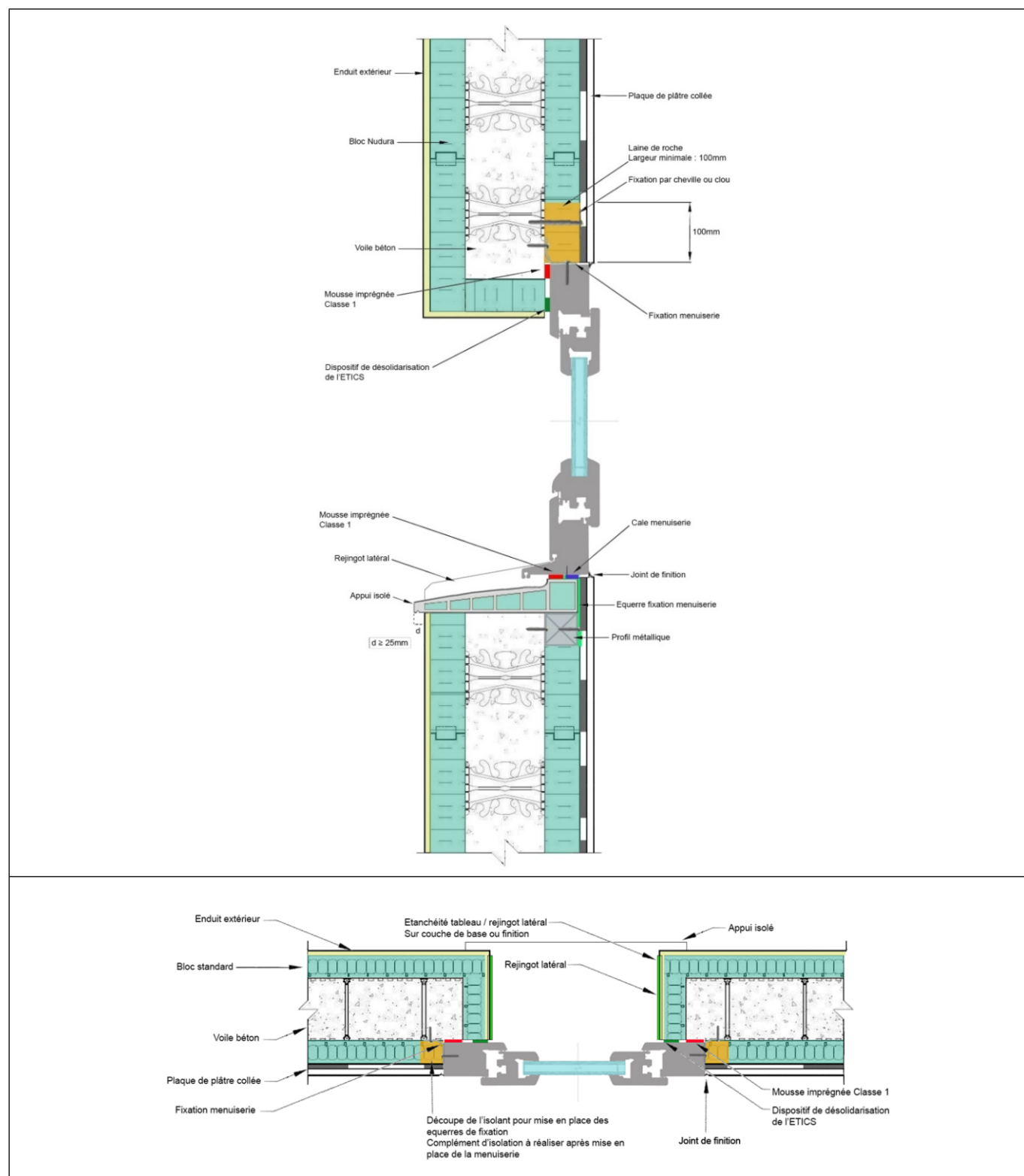
Figure 23 - Pose de menuiserie bois en applique (Finition avec plaques de plâtre collées)
