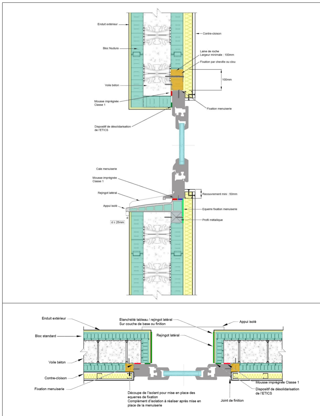
Figure 24 - Pose de menuiserie bois en applique (Finition avec contre-cloison et plaques de plâtre)
