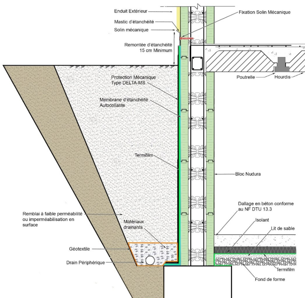
Figure 37 - Prévention contre les termites – Périphérie sous-sol dallage isolé en sous face et non porté
