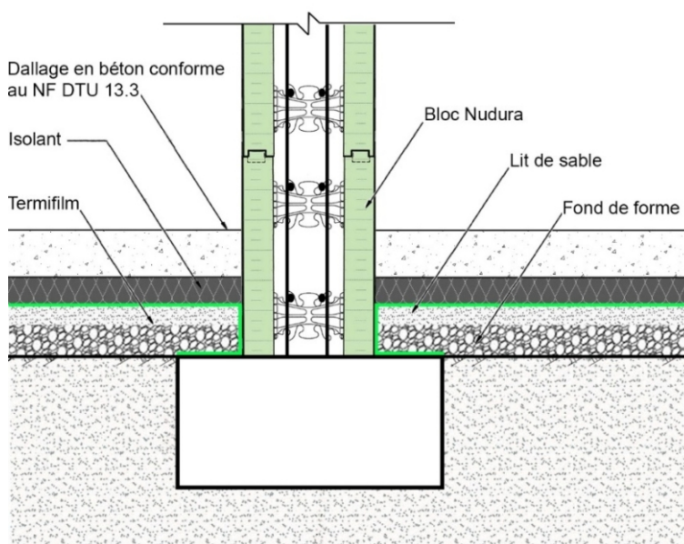
Figure 32 - Prévention contre les termites – Refend dallage sur terre-plein isolé en sous face et non porté
