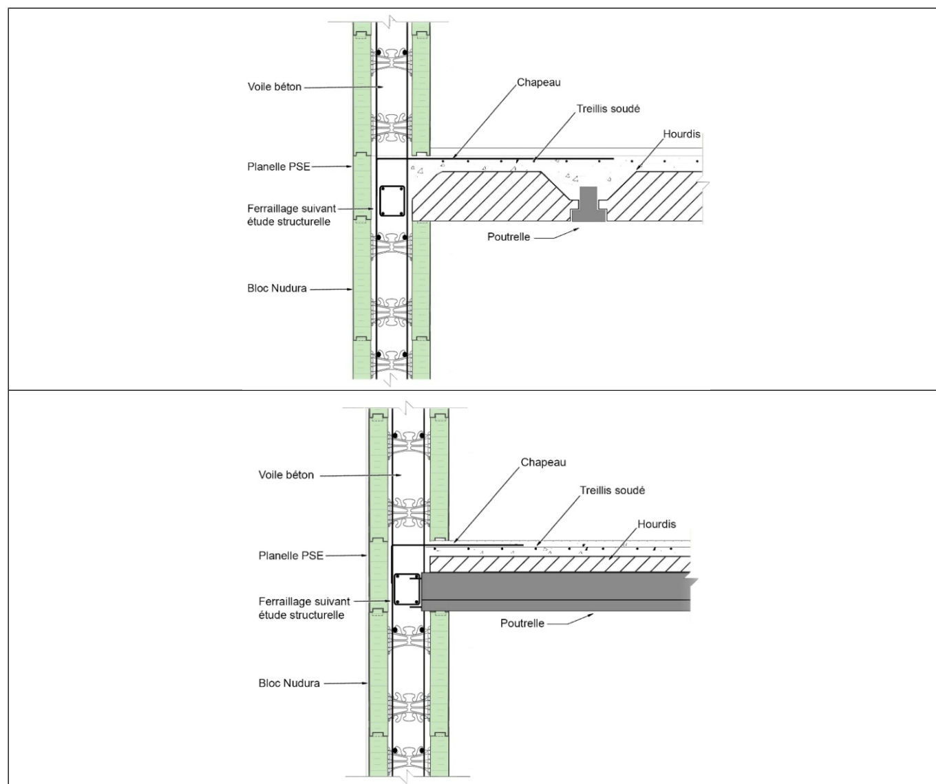
Figure 18 - Traitement des jonctions Mur Nudura / Planchers
