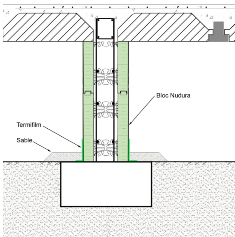
Figure 36 - Prévention contre les termites – Refend d'un vide sanitaire
