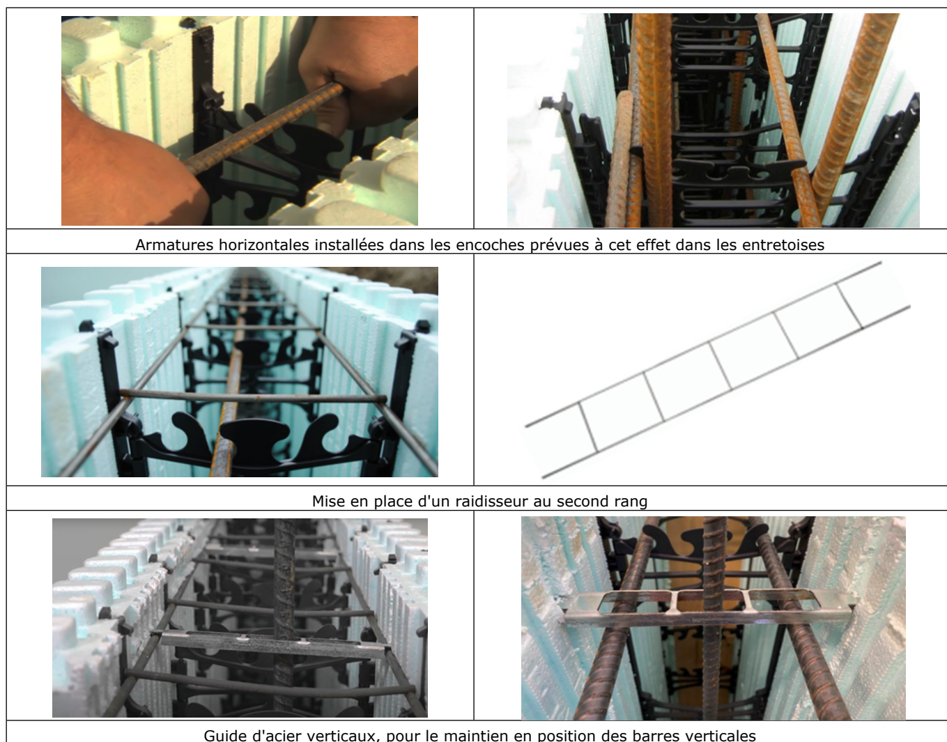
Figure 13 – Mise en œuvre – mise en place des ferrailages
