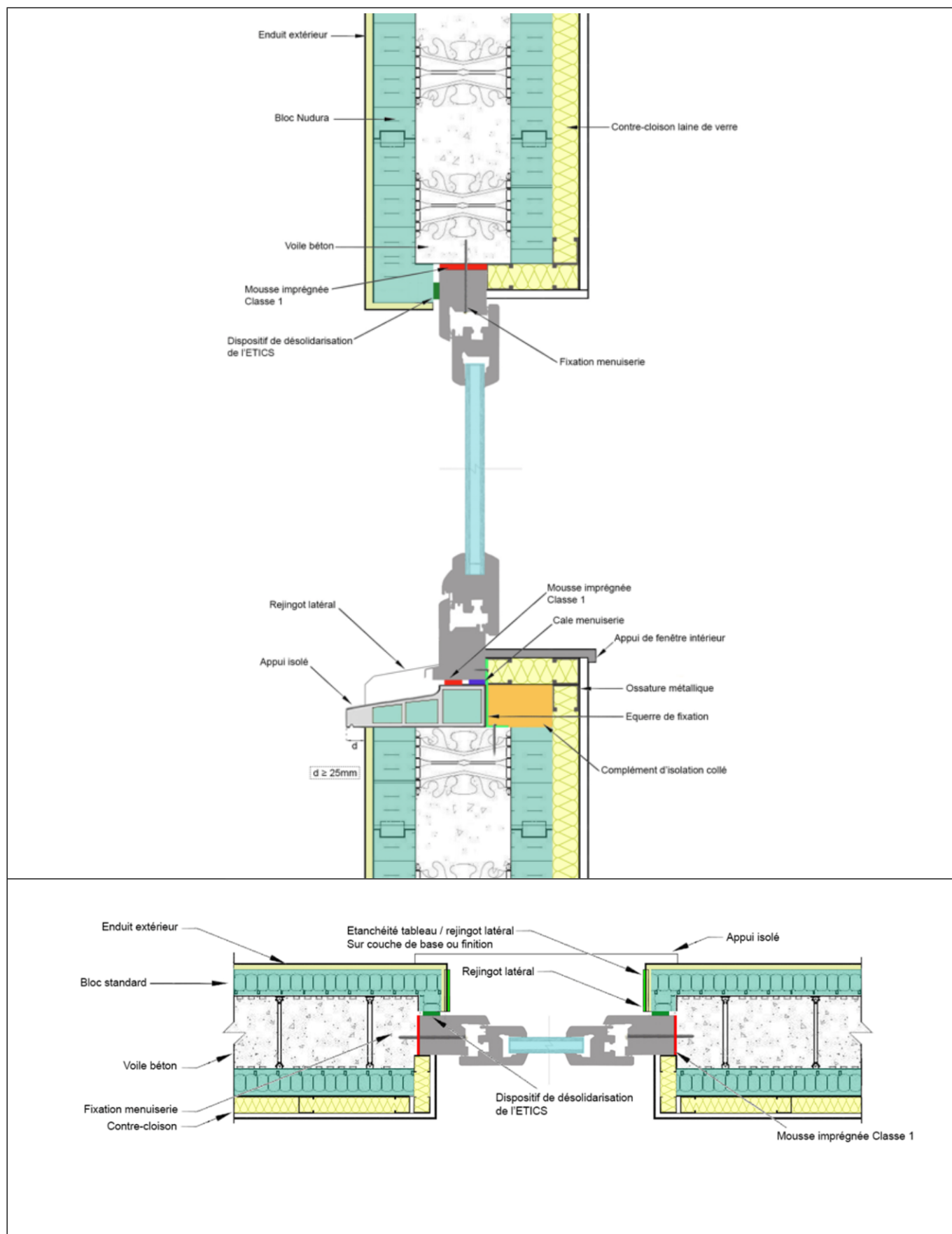
Figure 26 - Pose de menuiserie bois en tunnel (Finition avec contre-cloison et plaques de plâtre)
