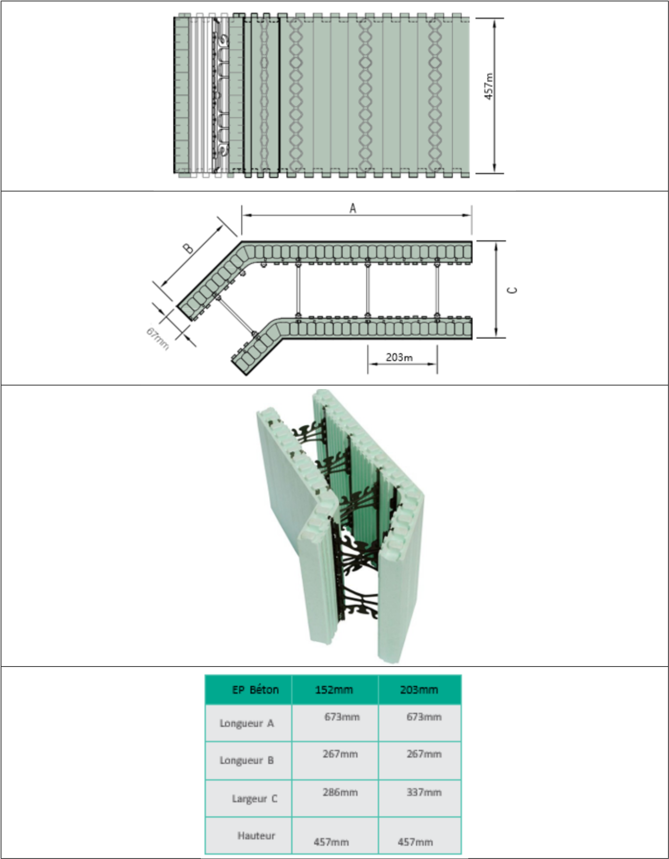
Figure 7 - Bloc d'angle 45° ICF
