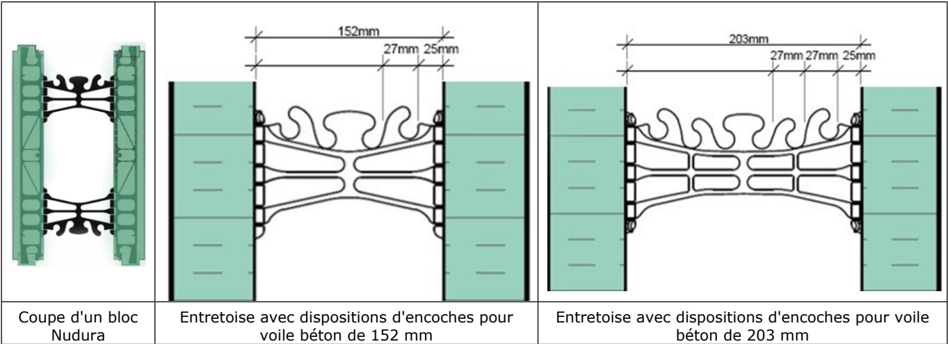
Figure 4 - Coupe d'un bloc Nudura et entretoise
