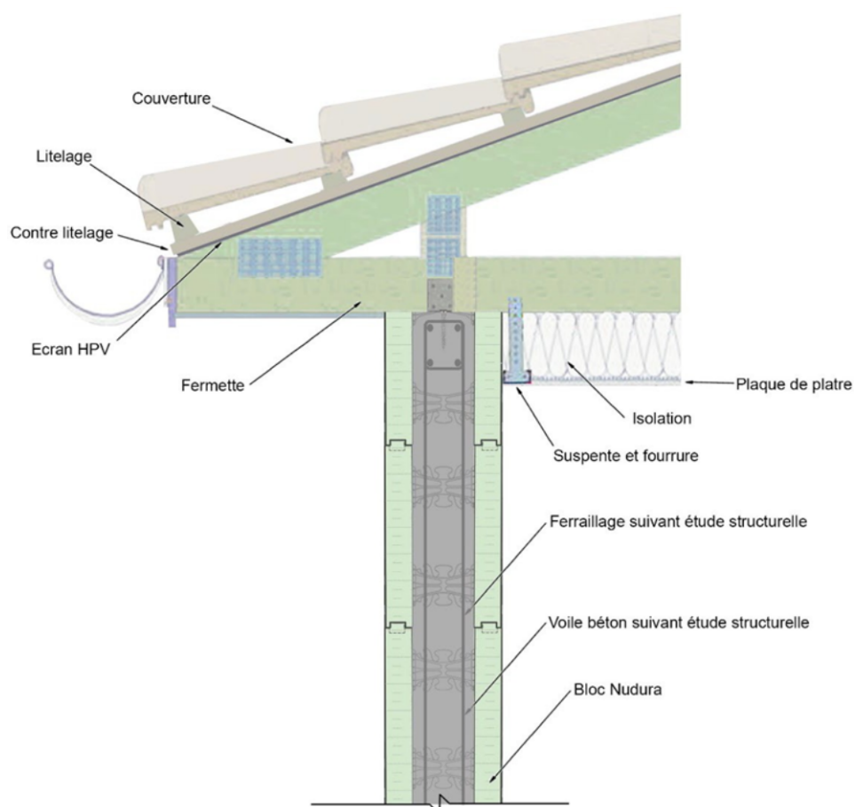
Figure 20 - Jonction Mur Nudura / Toiture (Charpente Fermettes)
