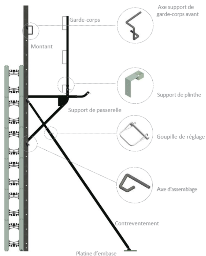
Figure 10 - Système d'étaie Nudura
