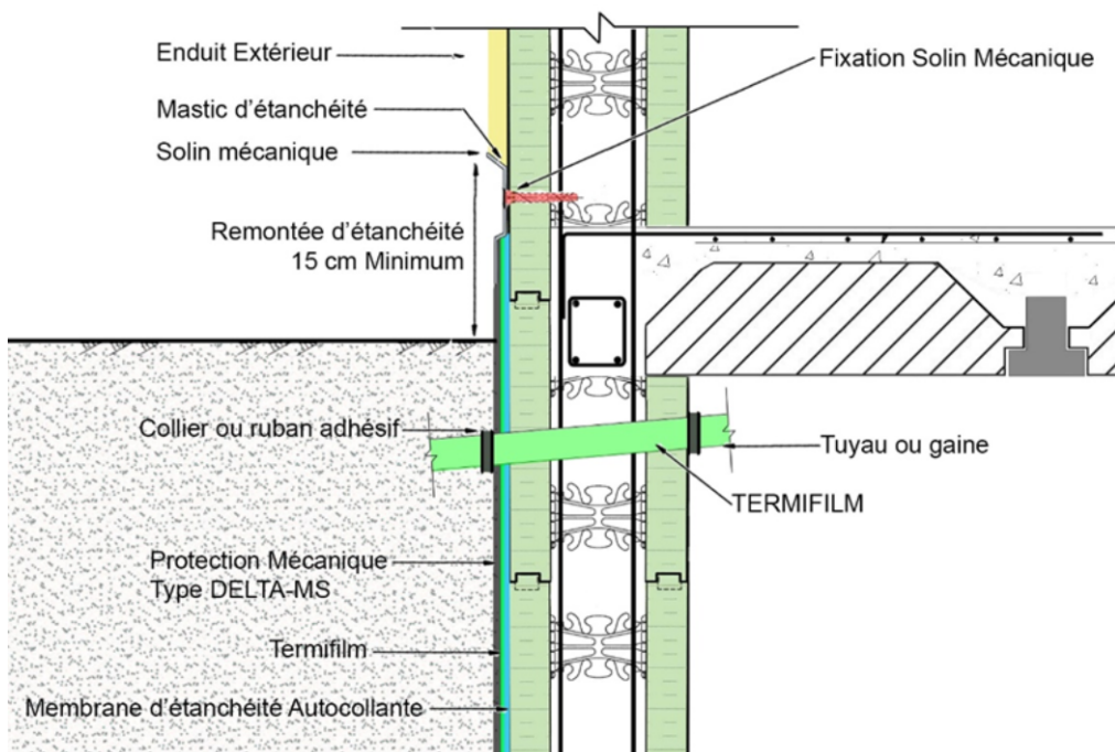
Figure 38 - Prévention contre les termites – Traitement des traversées avec film TERMIFILM
