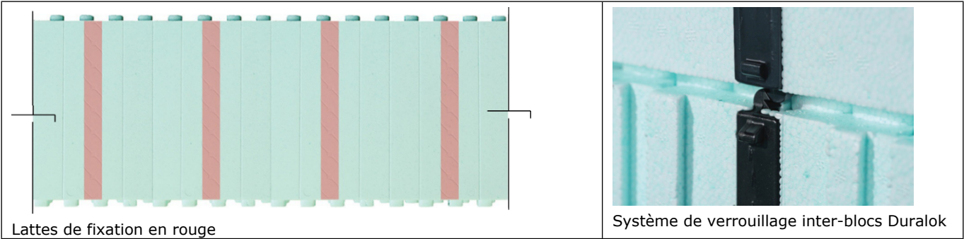
Figure 3 - Lattes de fixation sur face externe des planelles et système de verrouillage inter-blocs Duralok
