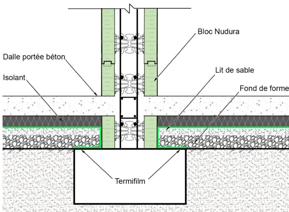
Figure 34 - Prévention contre les termites – Dallage sur terre-plein isolé et porté
