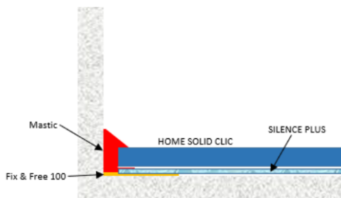
Figure 1 : Traitement des coupes et des joints périphériques dans le cas des locaux E2 et sur supports contenant de l'amiante
