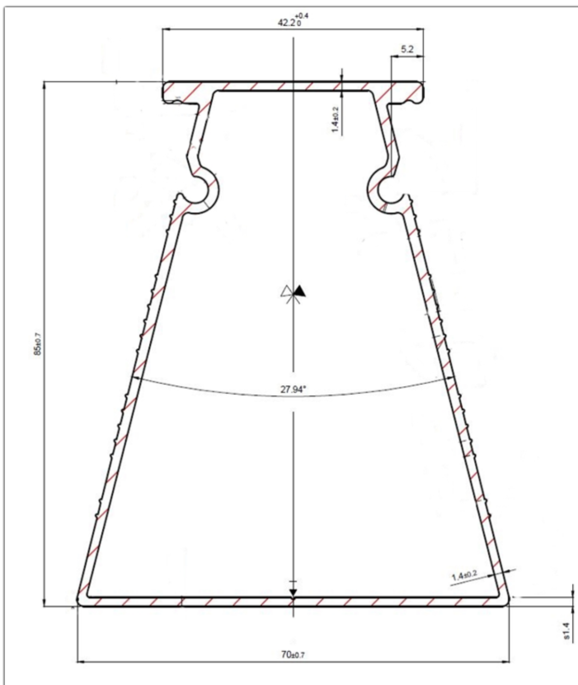
Figure 6 – Profil trapézoïdal
