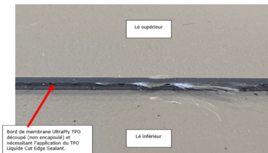
Figure 32 (suite) - Mise en œuvre du TPO Liquide Cut Edge Sealant
