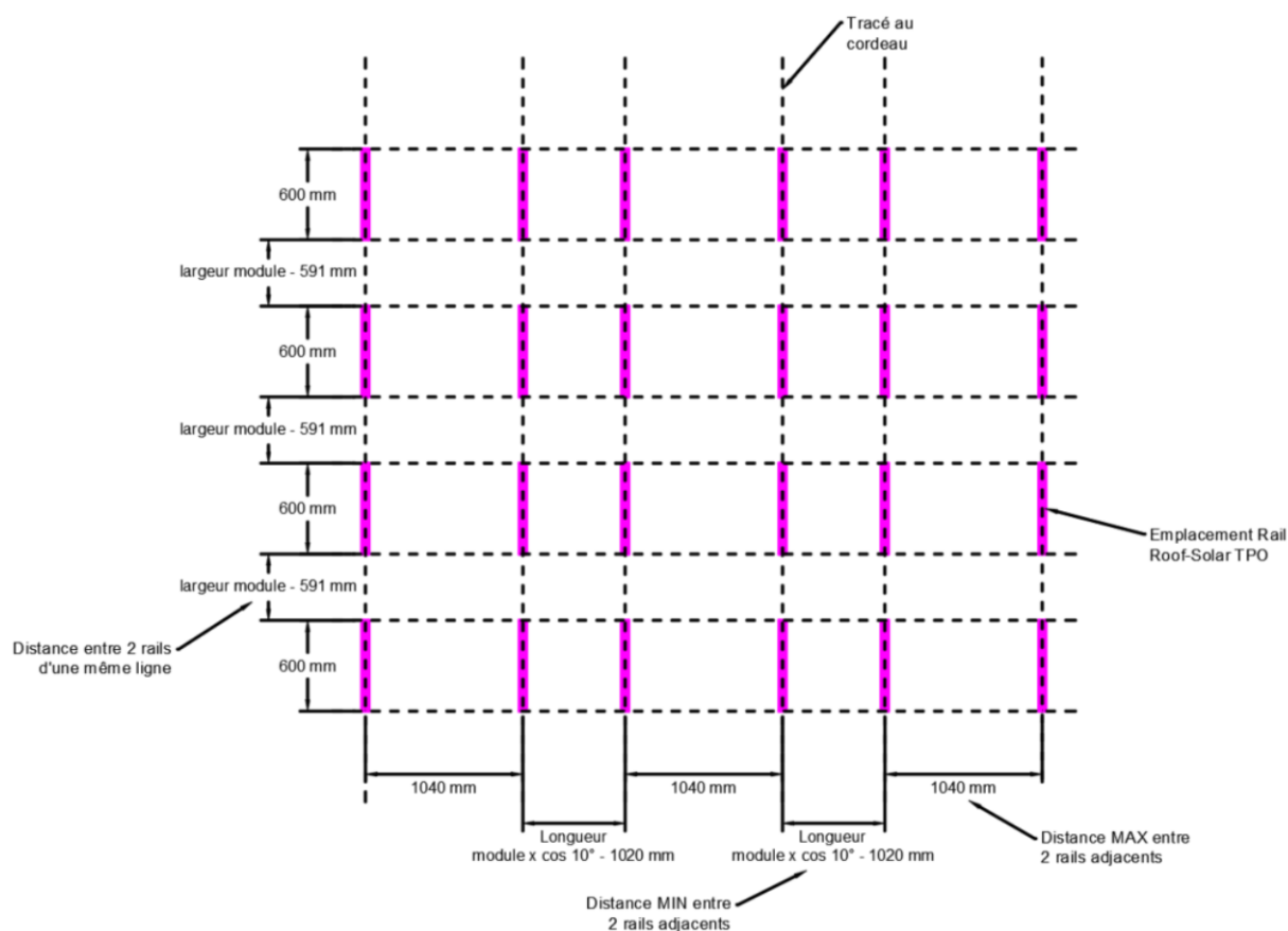
Figure 38 - Traçage des rails avec pose des modules en incliné simple shed
