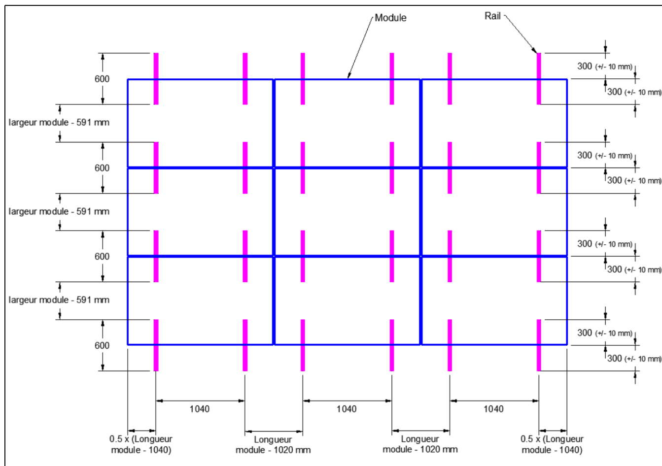
Figure 40 - Implantation des ensembles « Rail » / modules à plat
