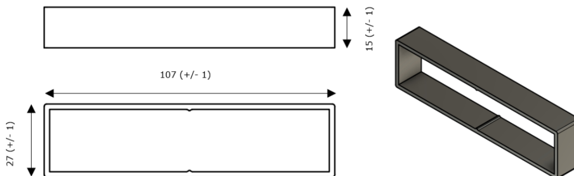
Figure 21 - Cale rotule du kit d'inclinaison du procédé ROOF-SOLAR TPO TAN DTU – Plat & Incliné
