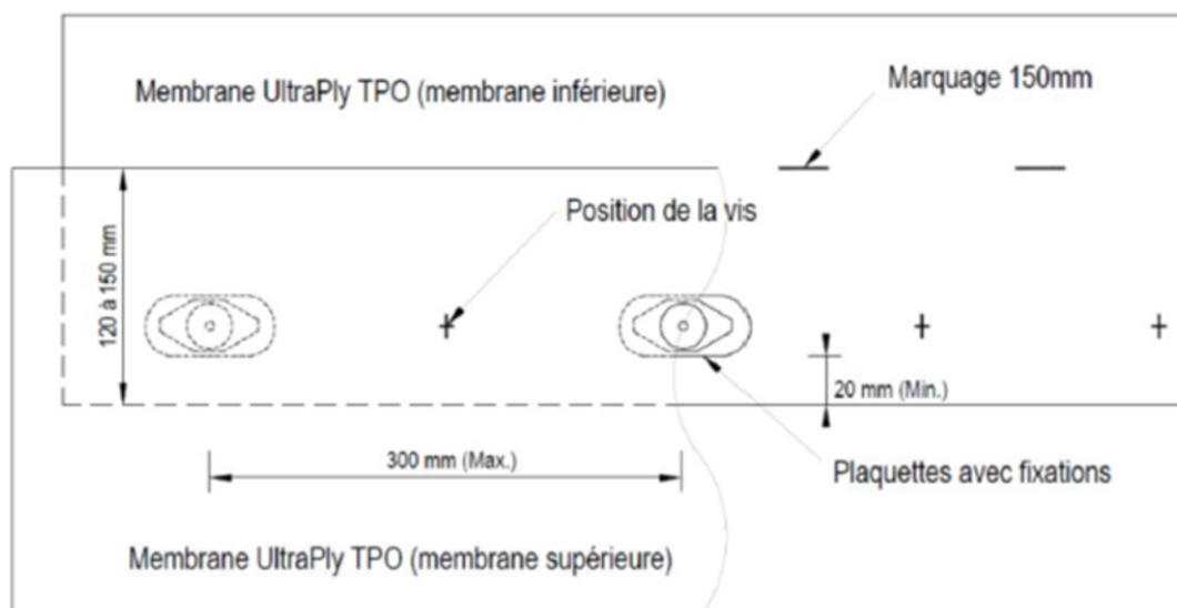
Fixation mécanique
