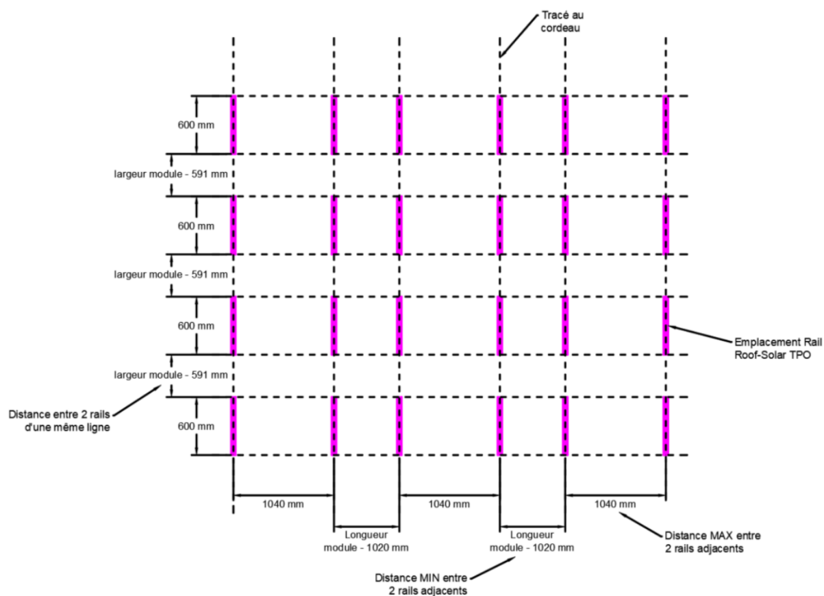
Figure 37 - Traçage des rails avec pose des modules à plat
