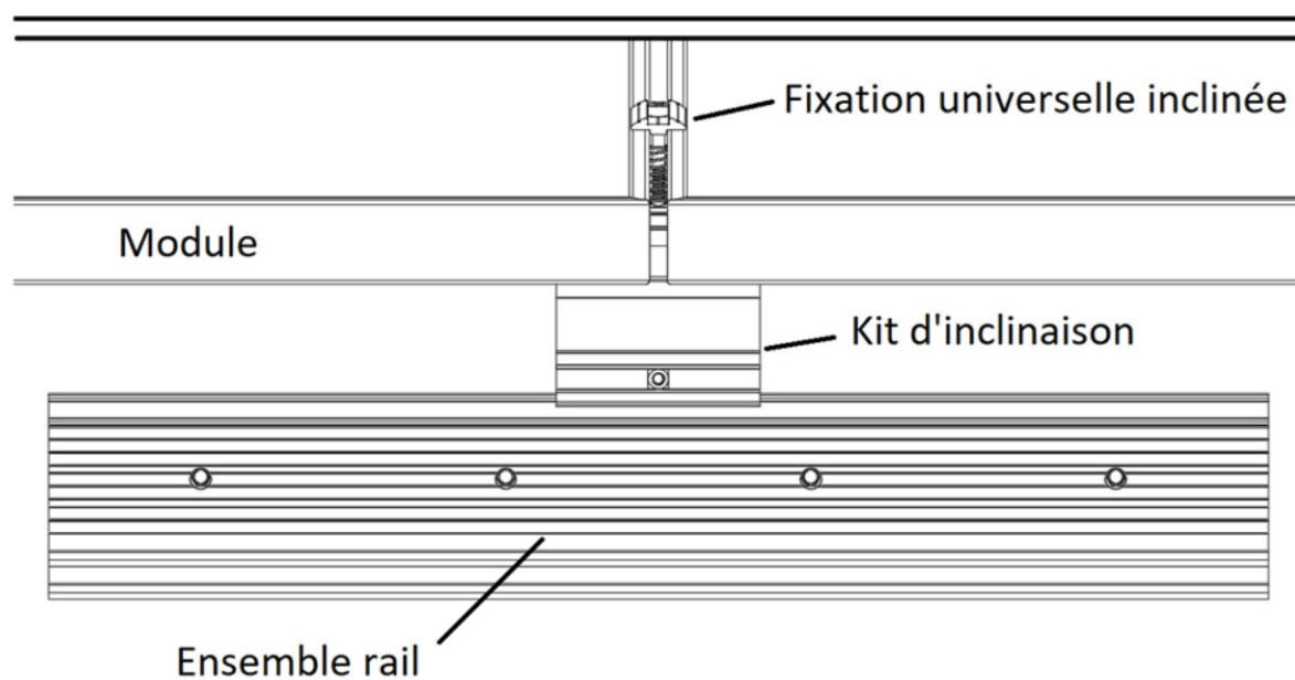
Figure35 (suite) - Assemblage rail / kit d'inclinaison / module
