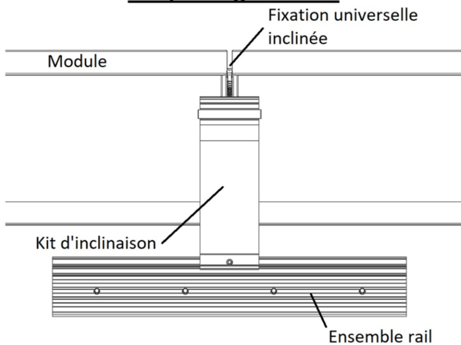
Figure 35 - Assemblage rail / kit d'inclinaison / module
