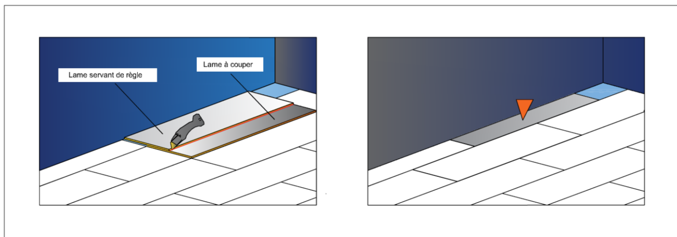
Figure 2 : découpe en périphérie par report
