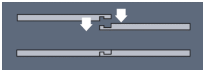
Figure 3 – Emboîtement du petit côté : clic à plat
