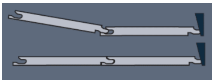
Figure 4 – Emboîtement du grand côté : clic angulaire
