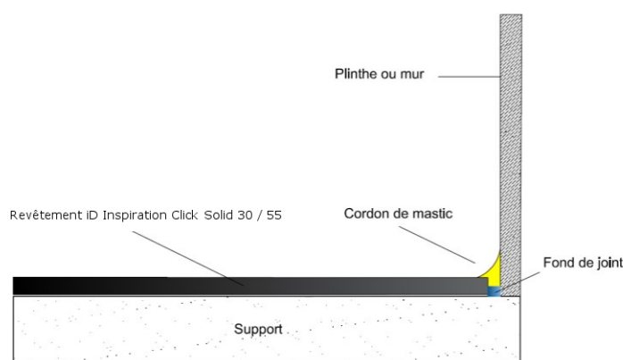
Figure 6 : Fond de joint et mastic (cas des locaux E2 y compris sur support contenant de l'amiante)
