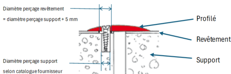
Figure 5 : Exemple de traitement des joints de dilatation du support avec profilés tels que décrits en Annexe 1.
