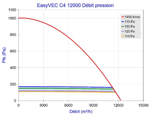
Figure 58 – EasyVEC C4 12 0000 (avec ou sans T.Flow Hygro+/T.Flow Nano ou T.Flow 105 / T.Flow 180)
