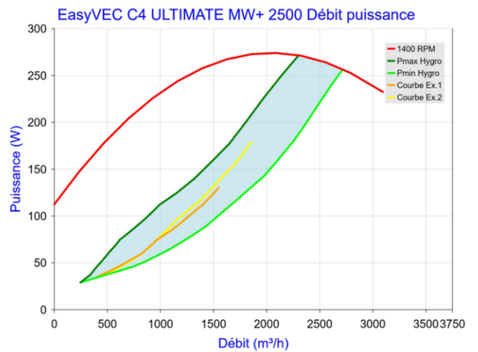
Figure 103 - EasyVEC C4 ULTIMATE MW+ 2500 (sans T.Flow Hygro+/T.Flow Nano ou T.Flow 105 / T.Flow 180)
