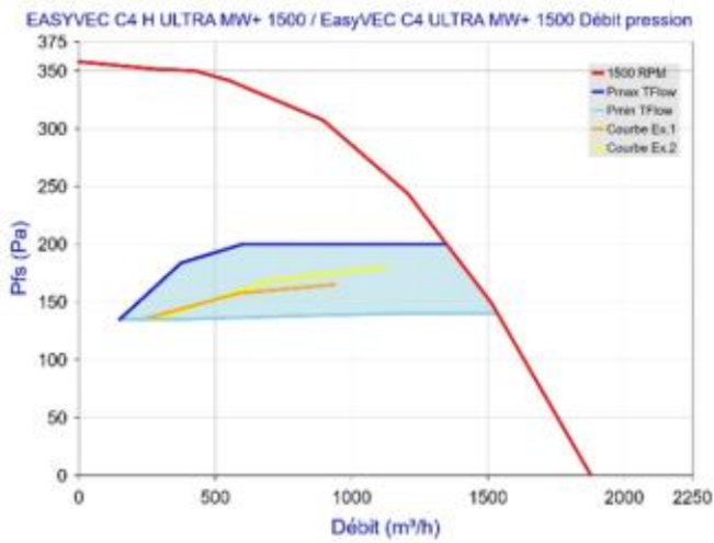
Figure 93 - EasyVEC C4 (H) ULTRA MW+ 1500 avec T.Flow Hygro+/T.Flow Nano ou T.Flow 105 / T.Flow 180
