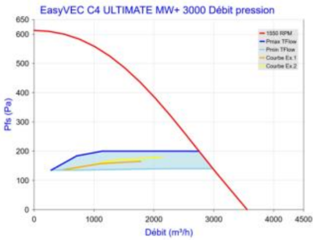
Figure 112 - EasyVEC C4 ULTIMATE MW+ 3000 avec T.Flow Hygro+/T.Flow Nano ou T.Flow 105 / T.Flow 180
