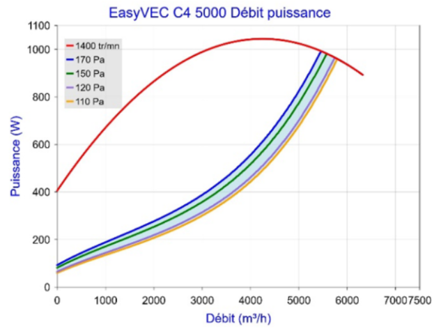
Figure 54 – EasyVEC C4 5000 (avec ou sans T.Flow Hygro+/T.Flow Nano ou T.Flow 105 / T.Flow 180)
