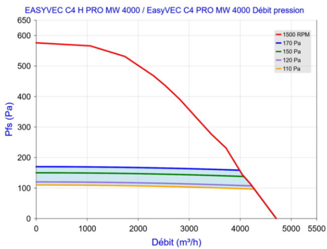
Figure 81 – EasyVEC C4 (H) PRO MW 4000 (avec ou sans T.Flow Hygro+/T.Flow Nano ou T.Flow 105 / T.Flow 180)
