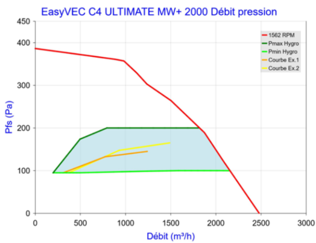
Figure 102- EasyVEC C4 ULTIMATE MW+ 2000 (sans T.Flow Hygro+/T.Flow Nano ou T.Flow 105 / T.Flow 180)
