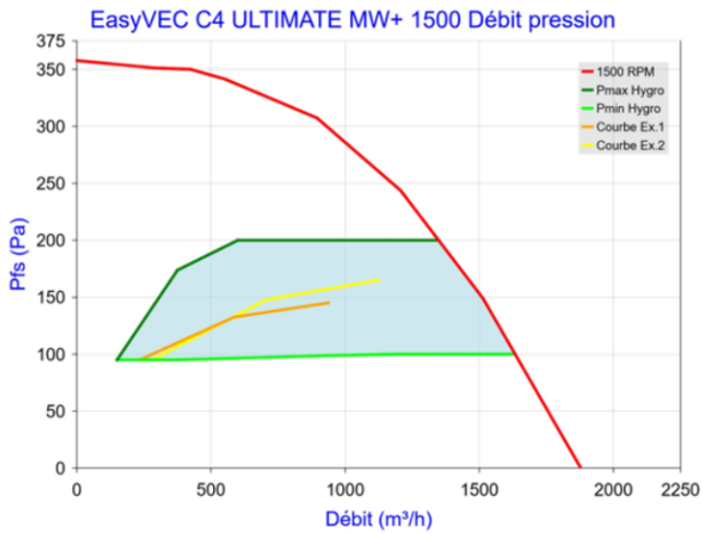
Figure 101 - EasyVEC C4 ULTIMATE MW+ 1500 (sans T.Flow Hygro+/T.Flow Nano ou T.Flow 105 / T.Flow 180)
