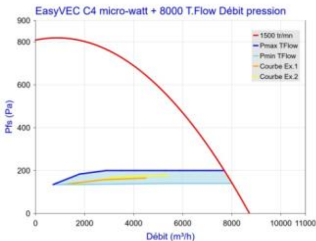
Figure 71 - EasyVEC C4 micro-watt + 8000 avec T.Flow Hygro+ / T.Flow Nano ou T.Flow 105 / T.Flow 180
