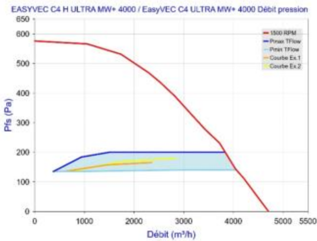
Figure 97 - EasyVEC C4 (H) ULTRA MW+ 4000 avec T.Flow Hygro+/ T.Flow Nano ou T.Flow 105 / T.Flow 180
