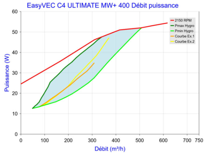
Figure 98 - EasyVEC C4 ULTIMATE MW+ 400 (sans T.Flow Hygro+/T.Flow Nano ou T.Flow 105 / T.Flow 180)
