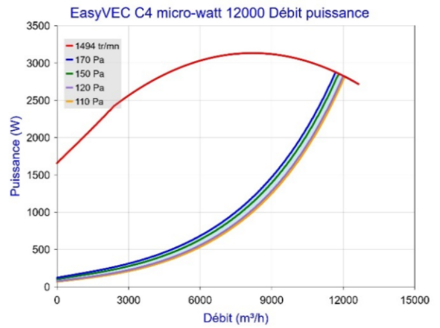
Figure 63 – EasyVEC C4 micro-watt 12000 (avec ou sans T.Flow Hygro+/T.Flow Nano ou T.Flow 105 / T.Flow 180)
