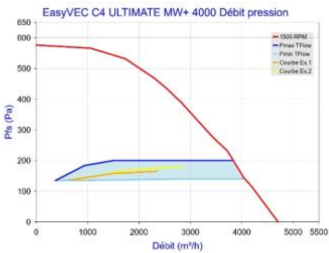
Figure 113 - EasyVEC C4 ULTIMATE MW+ 4000 avec T.Flow Hygro+/T.Flow Nano ou T.Flow 105 / T.Flow 180
