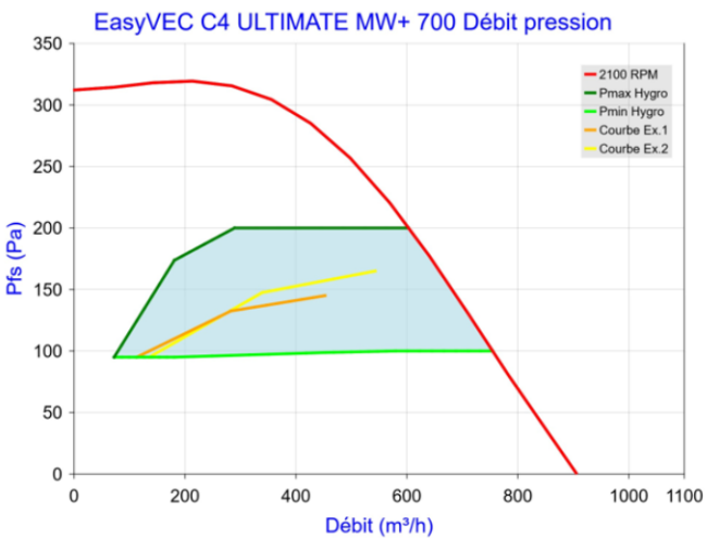
Figure 99 - EasyVEC C4 ULTIMATE MW+ 700 (sans T.Flow Hygro+/T.Flow Nano ou T.Flow 105 / T.Flow 180)
