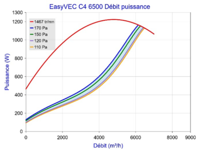
Figure 55 – EasyVEC C4 6500 (avec ou sans T.Flow Hygro+/T.Flow Nano ou T.Flow 105 / T.Flow 180)
