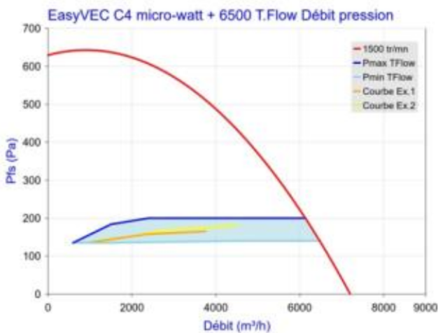
Figure 70 - EasyVEC C4 micro-watt + 6500 avec T.Flow Hygro+ / T.Flow Nano ou T.Flow 105 / T.Flow 180
