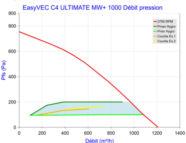
Figure 100 - EasyVEC C4 ULTIMATE MW+ 1000 (sans T.Flow Hygro+/T.Flow Nano ou T.Flow 105 / T.Flow 180)
