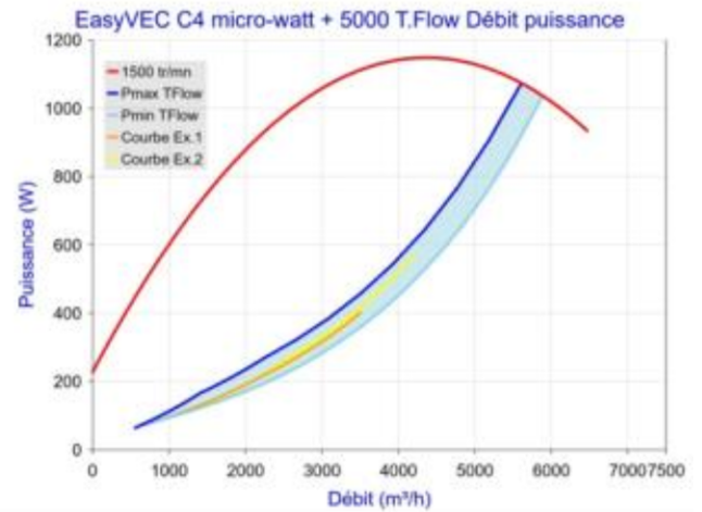
Figure 69 - EasyVEC C4 micro-watt + 5000 avec T.Flow Hygro+ / T.Flow Nano ou T.Flow 105 / T.Flow 180
