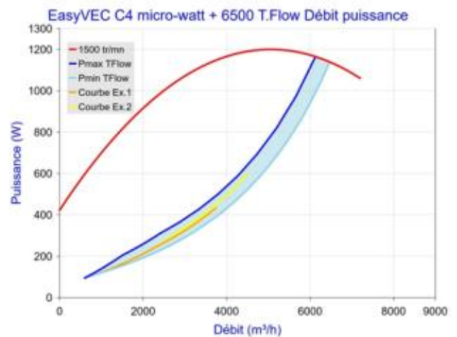
Figure 70 - EasyVEC C4 micro-watt + 6500 avec T.Flow Hygro+ / T.Flow Nano ou T.Flow 105 / T.Flow 180
