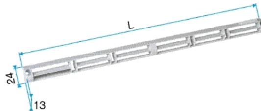
Figure 15 - Auvent standard pour mini EA 30 [2]
