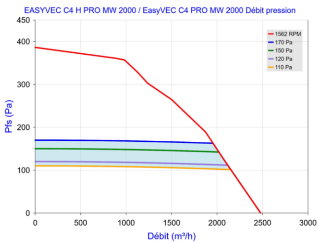
Figure 78 – EasyVEC C4 (H) PRO MW 2000 (avec ou sans T.Flow Hygro+/T.Flow Nano ou T.Flow 105 / T.Flow 180)
