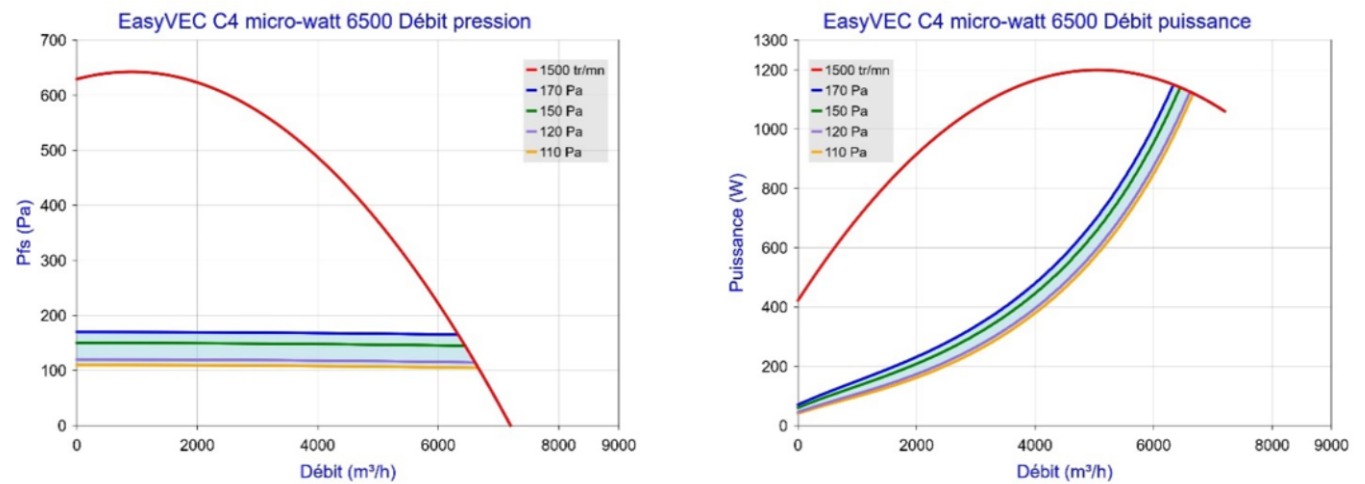
Figure 60 – EasyVEC C4 micro-watt 6500 (avec ou sans T.Flow Hygro+/T.Flow Nano ou T.Flow 105 / T.Flow 180)
