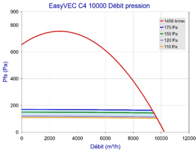
Figure 57 – EasyVEC C4 10000 (avec ou sans T.Flow Hygro+/T.Flow Nano ou T.Flow 105 / T.Flow 180)
