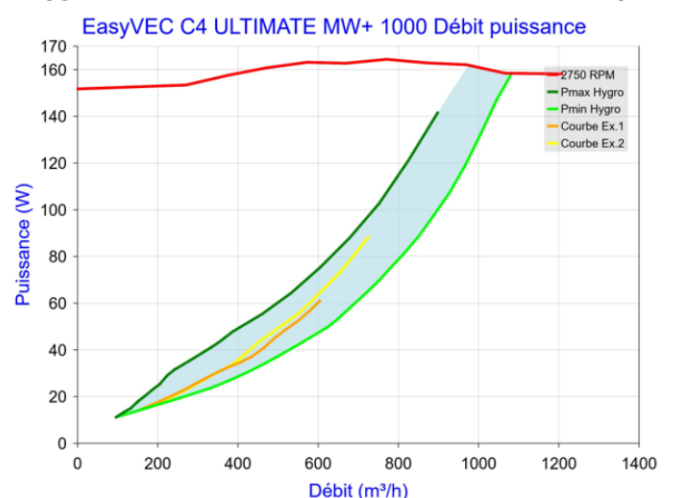
Figure 100 - EasyVEC C4 ULTIMATE MW+ 1000 (sans T.Flow Hygro+/T.Flow Nano ou T.Flow 105 / T.Flow 180)
