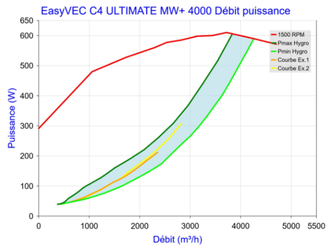
Figure 105 - EasyVEC C4 ULTIMATE MW+ 4000 (sans T.Flow Hygro+/T.Flow Nano ou T.Flow 105 / T.Flow 180)
