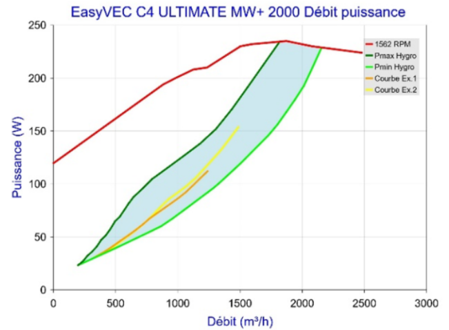
Figure 102- EasyVEC C4 ULTIMATE MW+ 2000 (sans T.Flow Hygro+/T.Flow Nano ou T.Flow 105 / T.Flow 180)
