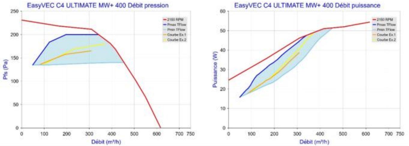
Figure 106 - EasyVEC C4 ULTIMATE MW+ 400 avec T.Flow Hygro+/T.Flow Nano ou T.Flow 105 / T.Flow 180
