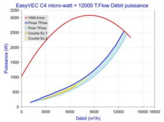
Figure 73 - EasyVEC C4 micro-watt + 12000 avec T.Flow Hygro+/ T.Flow Nano ou T.Flow 105 / T.Flow 180
