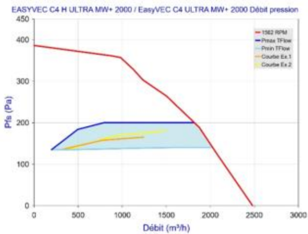
Figure 94 - EasyVEC C4 (H) ULTRA MW+ 2000 avec T.Flow Hygro+/ T.Flow Nano ou T.Flow 105 / T.Flow 180
