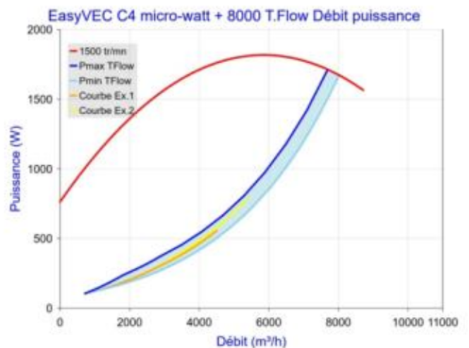
Figure 71 - EasyVEC C4 micro-watt + 8000 avec T.Flow Hygro+ / T.Flow Nano ou T.Flow 105 / T.Flow 180
