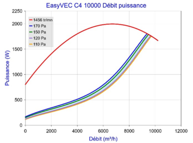
Figure 57 – EasyVEC C4 10000 (avec ou sans T.Flow Hygro+/T.Flow Nano ou T.Flow 105 / T.Flow 180)
