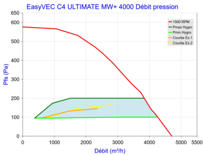
Figure 105 - EasyVEC C4 ULTIMATE MW+ 4000 (sans T.Flow Hygro+/T.Flow Nano ou T.Flow 105 / T.Flow 180)
