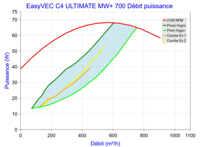
Figure 99 - EasyVEC C4 ULTIMATE MW+ 700 (sans T.Flow Hygro+/T.Flow Nano ou T.Flow 105 / T.Flow 180)
