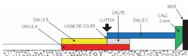
Figure 7 - Découpe par report
