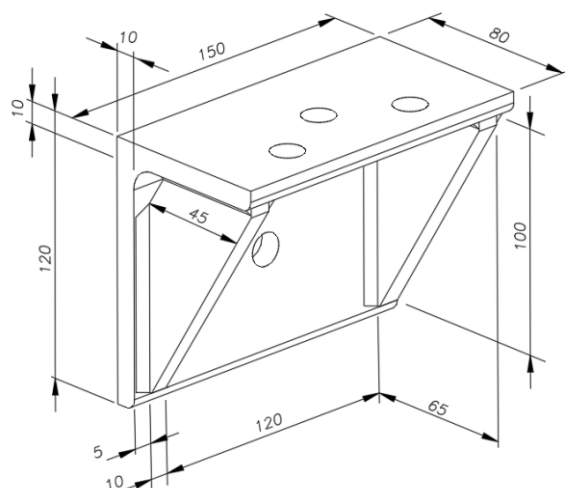
Figure 10 – Support d'équerre (Réf : 0070EQIN150)
