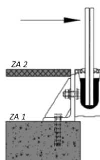
Pose latérale sur équerre
