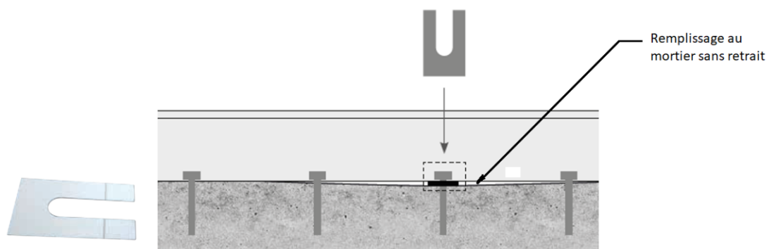
Figure 19 – Exemple de cale fourchette de calage sous le profil pour un montage sur du béton
