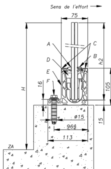
Référence de pose 7017 sur muret
