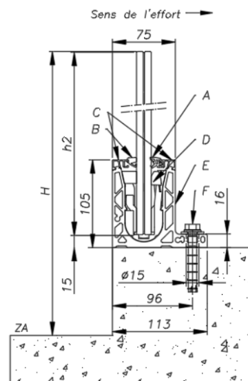
Référence de pose 7017R sur muret
