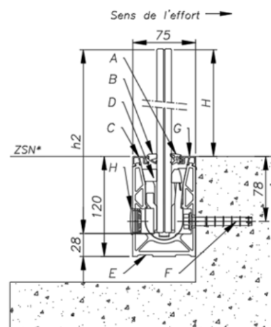
Référence de pose 7031R
