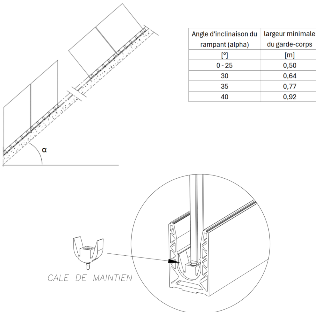
Figure 14 – Typologie des rampants
