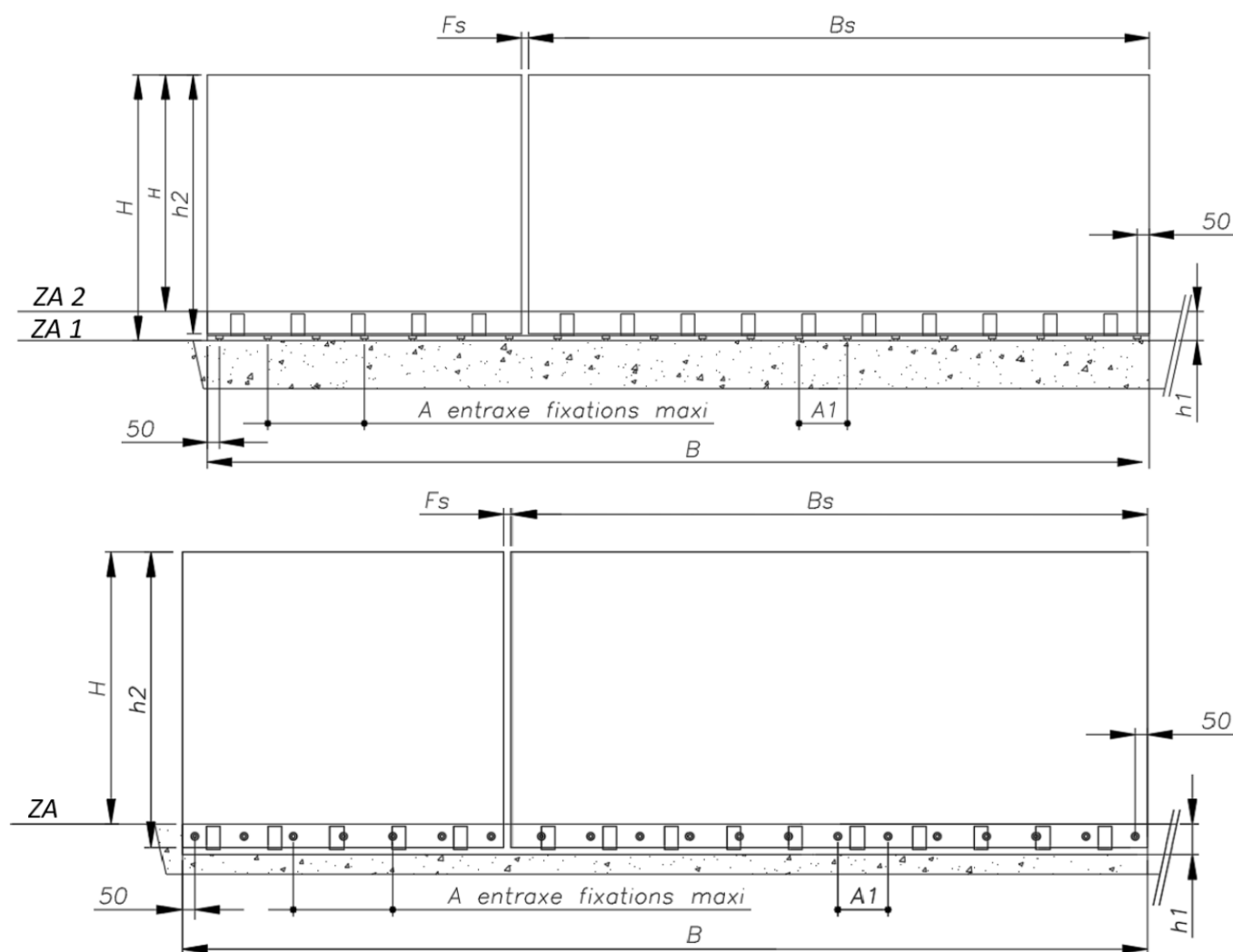
Figure 22 – Schéma dimensions des garde-corps (références de poses Tableau 16)
