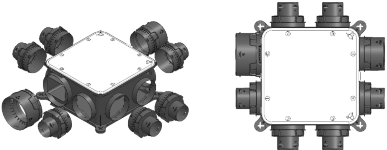
Figure 37b – Groupes d'extraction « MODULVENT HYGRO POWER-SAVE M » et « MODULVENT HYGRO POWER-SAVE L » - vue éclatée et vue de dessus du caisson + 1 adaptateur 160 mm + 1 adaptateur 125 mm + 6 adaptateurs 125/80 mm
