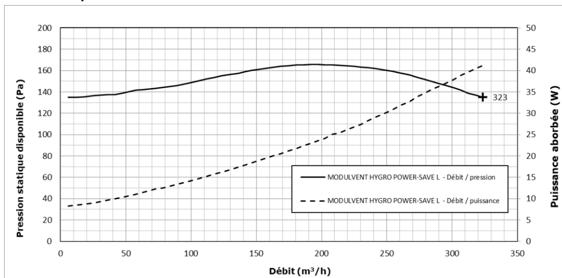
Figure 40 – Groupe d'extraction « MODULVENT HYGRO POWER-SAVE L » - courbes caractéristiques
