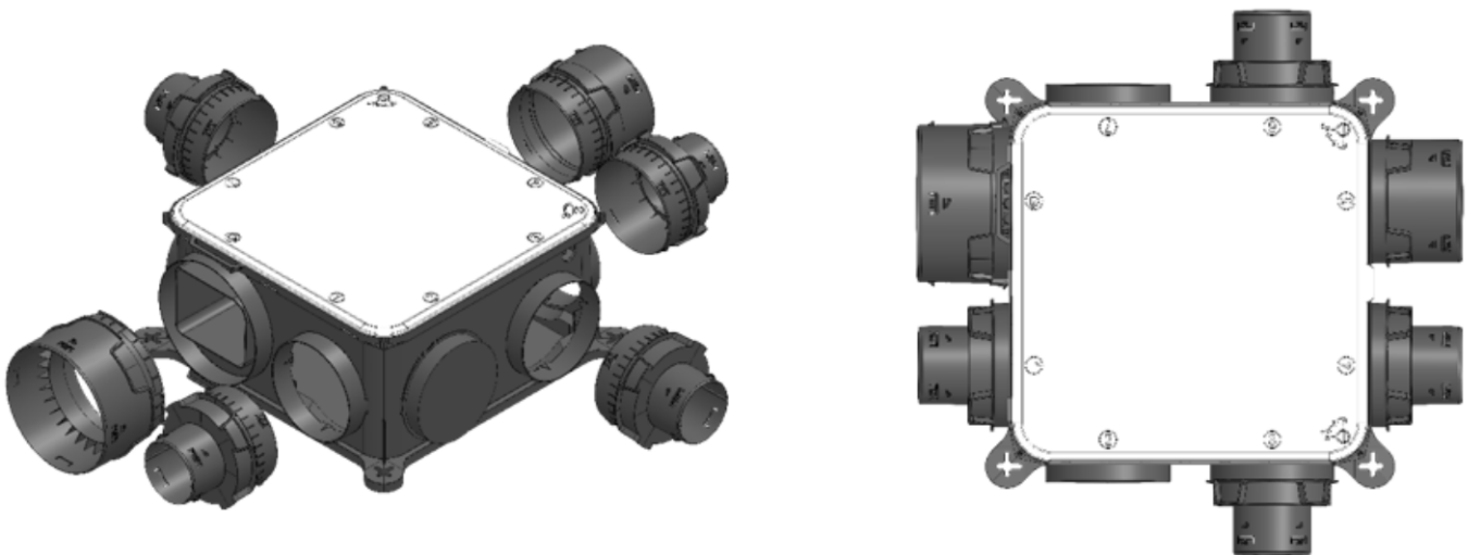
Figure 37a – Groupe d'extraction « MODULVENT HYGRO » - vue éclatée et vue de dessus du caisson + 1 adaptateur 160 mm + 1 adaptateur 125 mm + 4 adaptateurs 125/80 mm + 2 bouchons 125 mm
