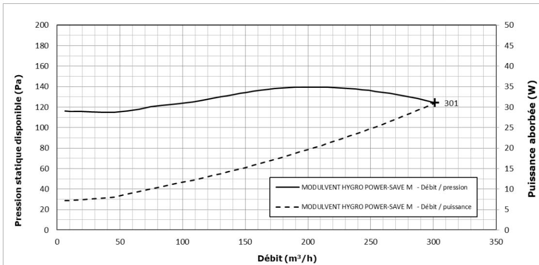
Figure 39 – Groupe d'extraction « MODULVENT HYGRO POWER-SAVE M » - courbes caractéristiques
