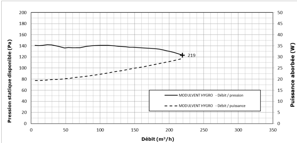
Figure 38 – Groupe d'extraction « MODULVENT HYGRO » - courbes caractéristiques
