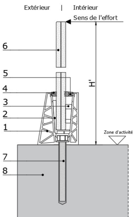
Figure 3 – GlassFit SV-1801 RX Top – Montage au sol
