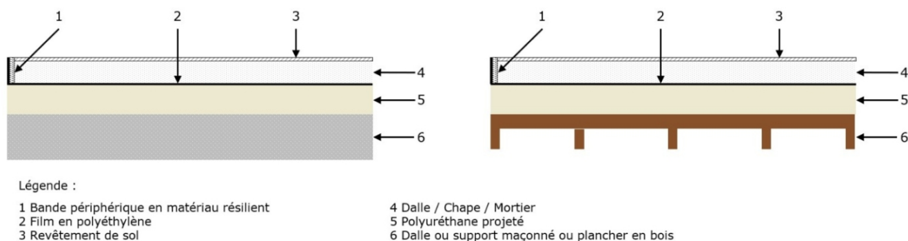
Figure 2 : Coupe avec support béton ou maçonnerie et plancher bois (schéma de principe)
