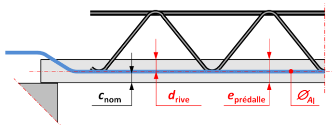
Figure 5 – Effort tranchant en rive – Définition des paramètres
