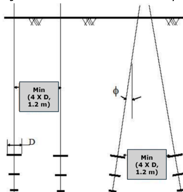
Figure 3 - Distance minimale d'installation des pieux
