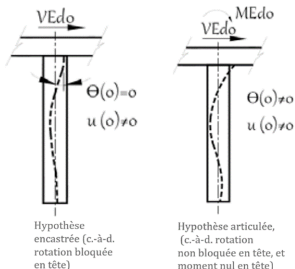
Figure 4 – Pieu encastré et articulé en tête
