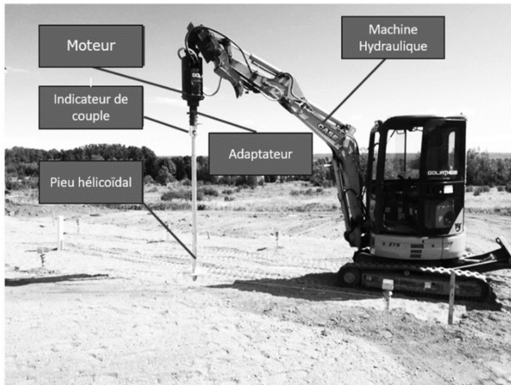
Figure 18 - Équipement typique d'installation de pieux hélicoïdaux
