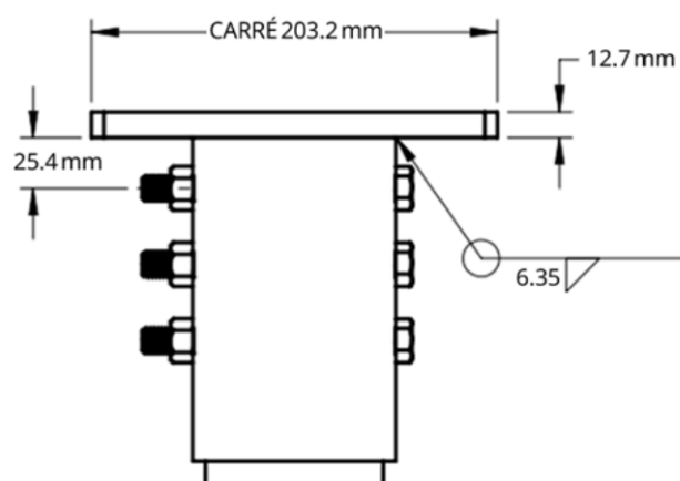
Figure 11 - Détail typique d'un support de tête du pieu hélicoïdal (support charpentes métallique et fondations superficielles en béton)
