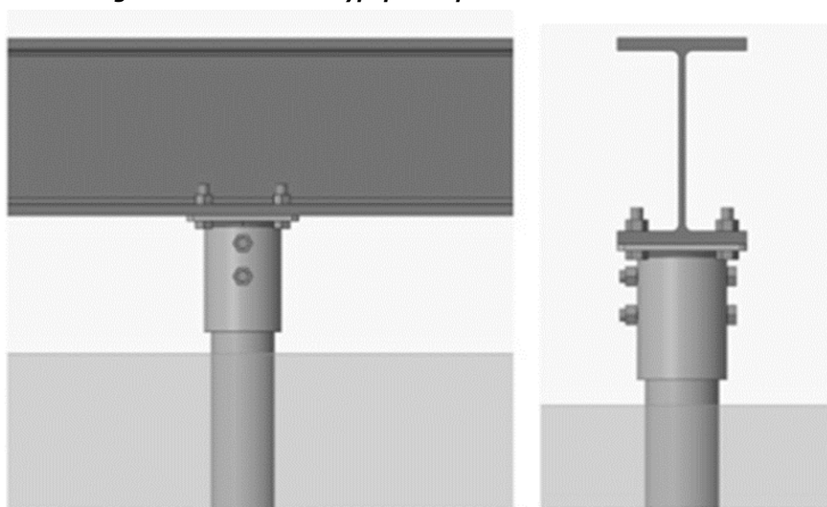
Figure 17 - Connexion typique du pieu à la structure en acier
