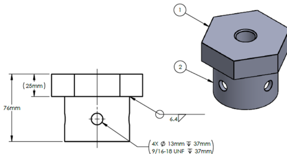
Figure 9 - Support typique ajustable/tête du pieu pour pieux hélicoïdaux (support charpentes métallique et bois)
