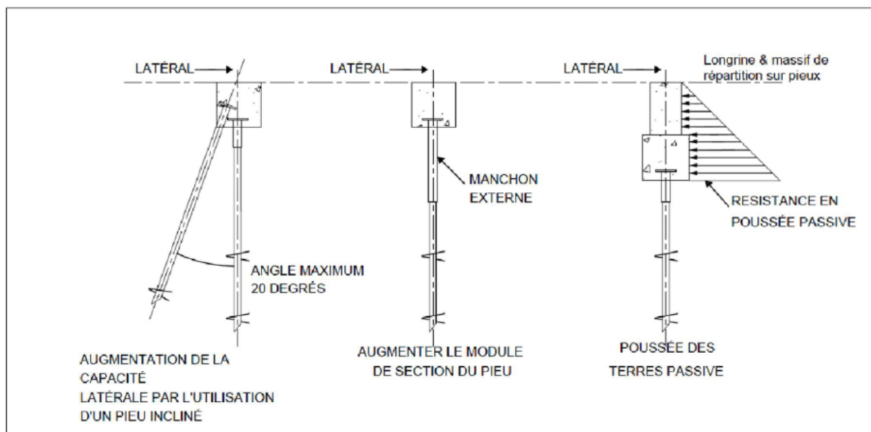
Figure 15 - Différentes manières d'augmenter la capacité latérale des pieux hélicoïdaux
