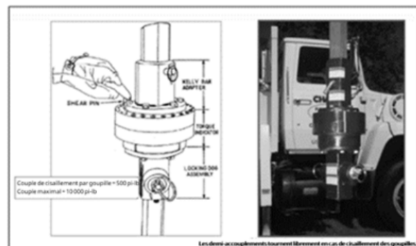
Figure 19 - Appareils de mesure de couple d'installation
