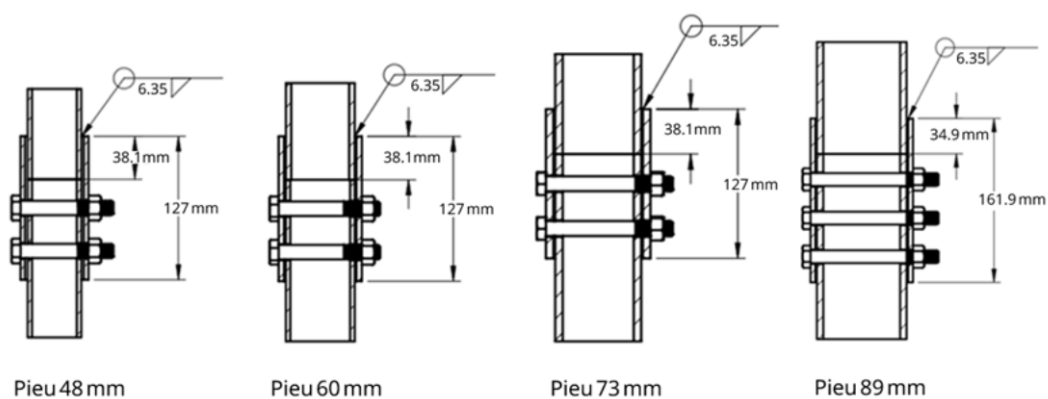
Figure 10 - Détail d'accouplement typique d'un pieu hélicoïdal
