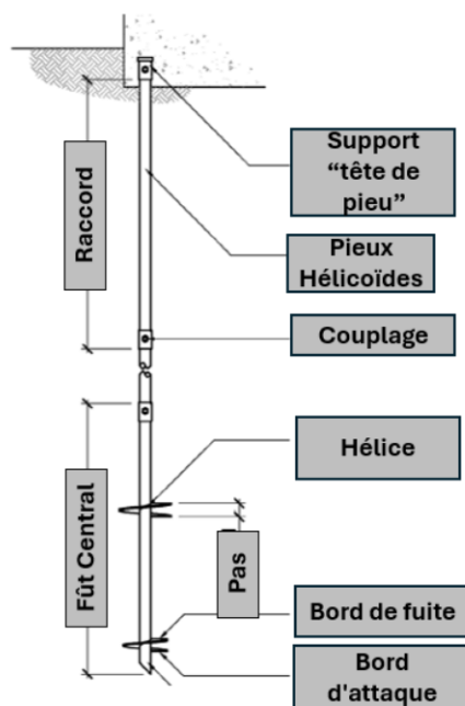
Figure 1 - Composants d'un pieu hélicoïdal
