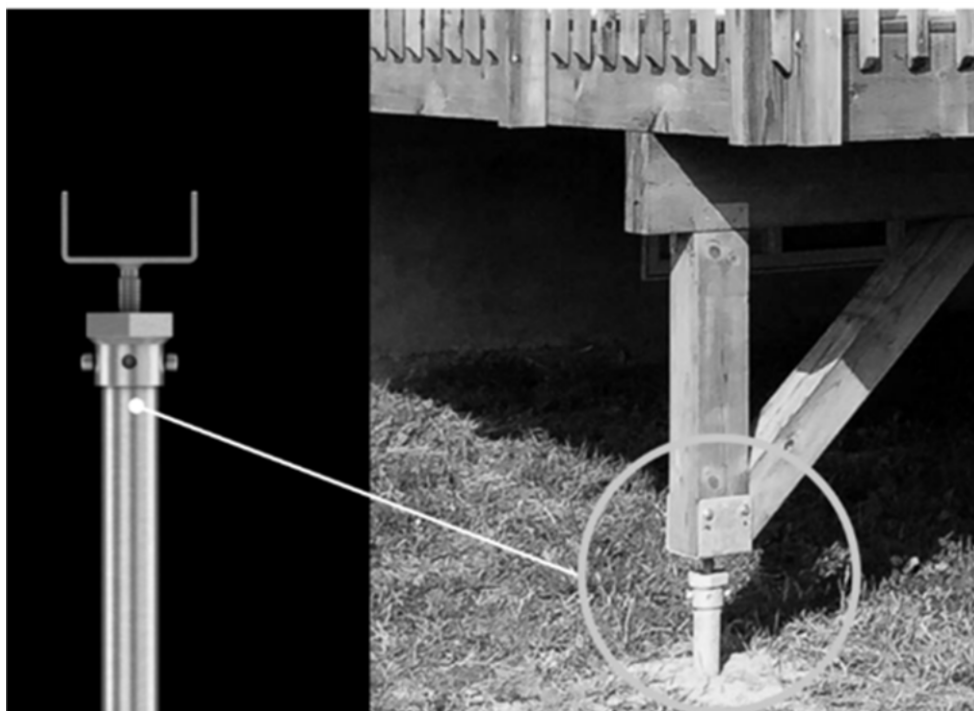
Figure 16 - Connexion typique du pieu à la structure en bois
