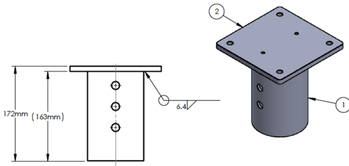
Figure 8 - Support/tête du pieu typique pour pieux hélicoïdaux (support charpentes métalliques et fondations superficielles en béton)
