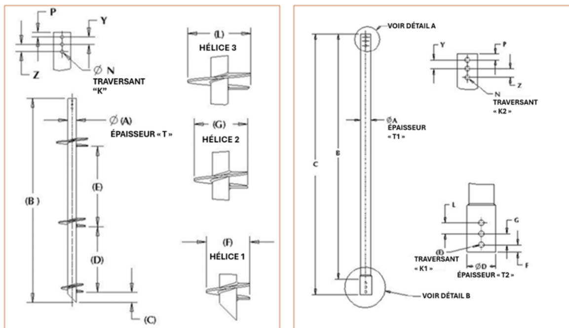
Figure 7 - Fut et Rallonge du Fut
