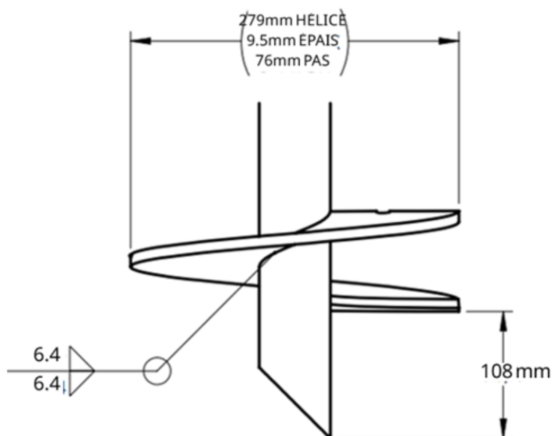
Figure 12 - Détail typique d'une hélice de pieu hélicoïdal
