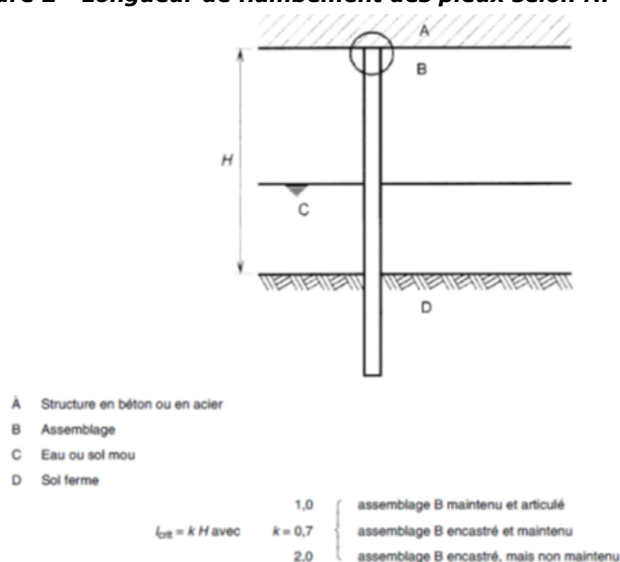
Figure 2 - Longueur de flambement des pieux selon NF EN 1997
