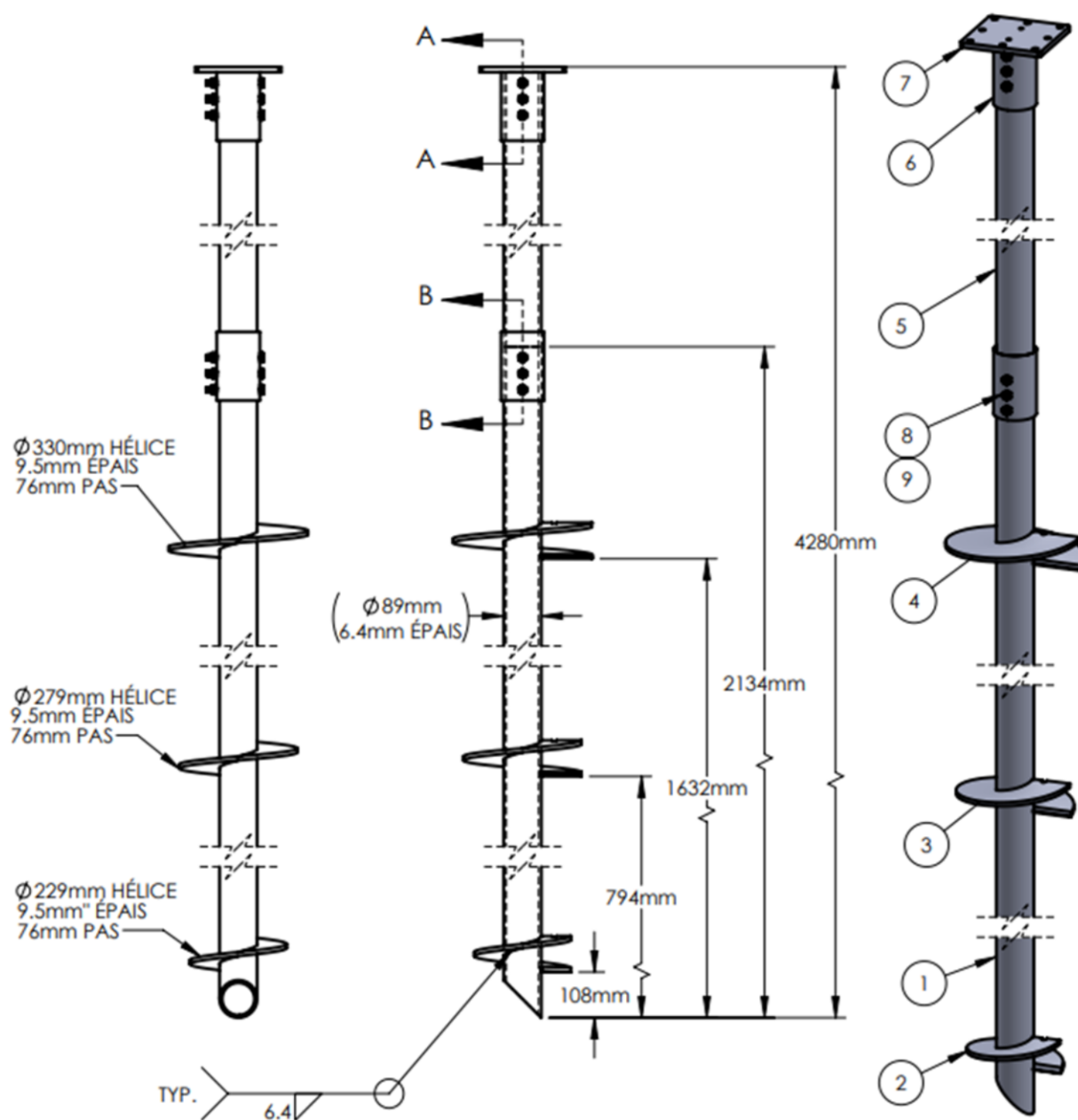
Figure 6 - Pieu hélicoïdale avec une rallonge et une configuration multi-hélice
