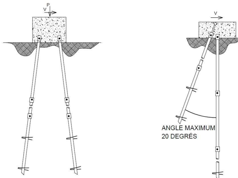
Figure 14 - Usage de piles hélicoïdales obliques pour augmenter la capacité latérale
